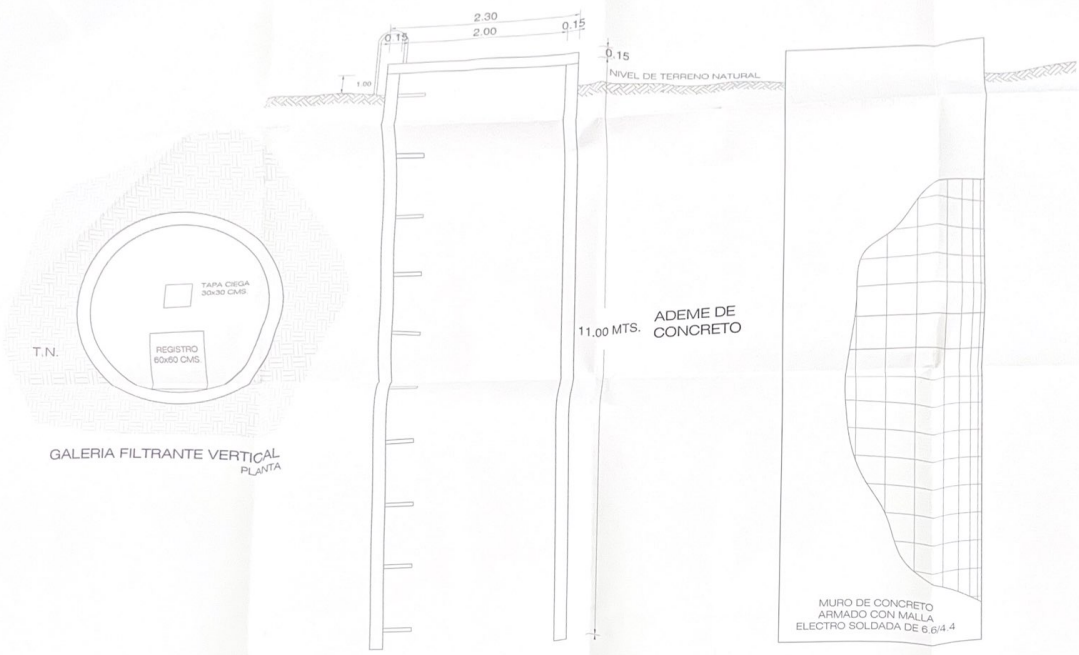
DETALLE DE ARMADO DE MURO FUERA DE ESCALA
