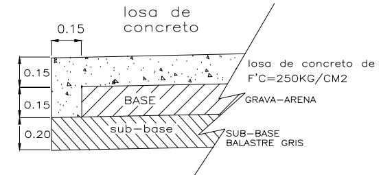
detalle constructivo en boca de calles y uniones de pavimentos
