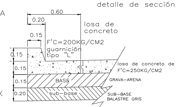
detalle constructivo
