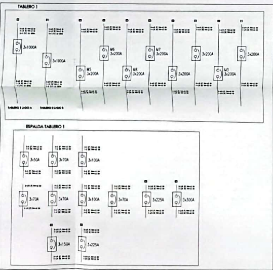
VISTAS FRONTALES DE TABLEROS EXISTENTES Y UBICACION EN CUARTO DE MAQUINAS
