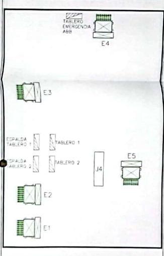
VISTAS FRONTALES DE TABLEROS EXISTENTES Y UBICACION EN CUARTO DE MAQUINAS
