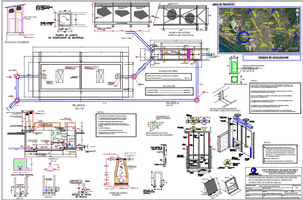
(anexo plano detalle de Caja de Retención)
