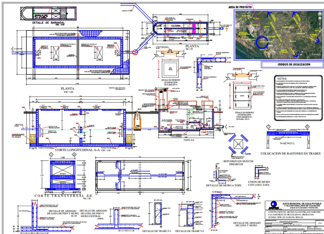
(anexo plano detalle de Fosa Septica)
