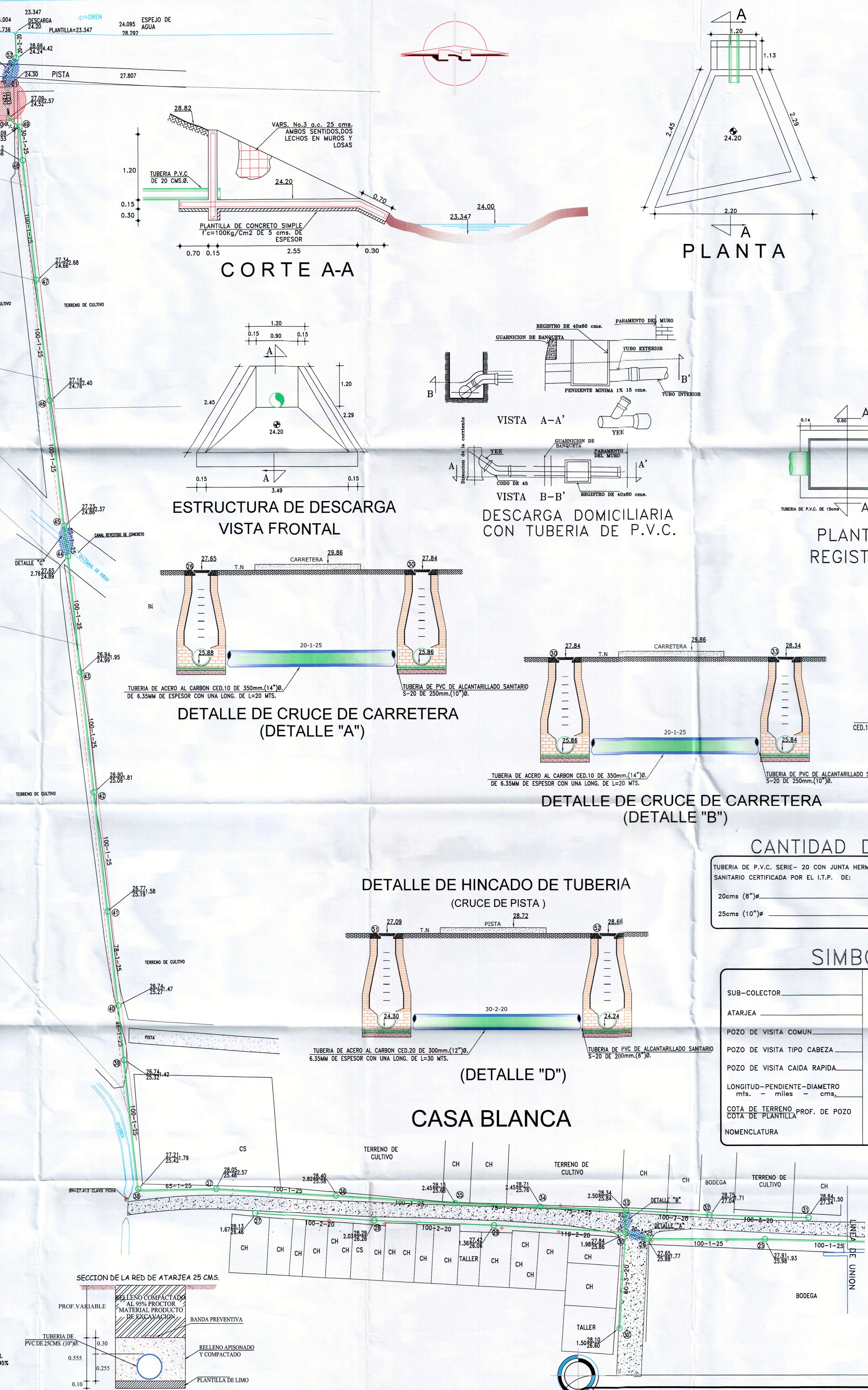
RED DE ALCANTARILLADO SANITARIO
