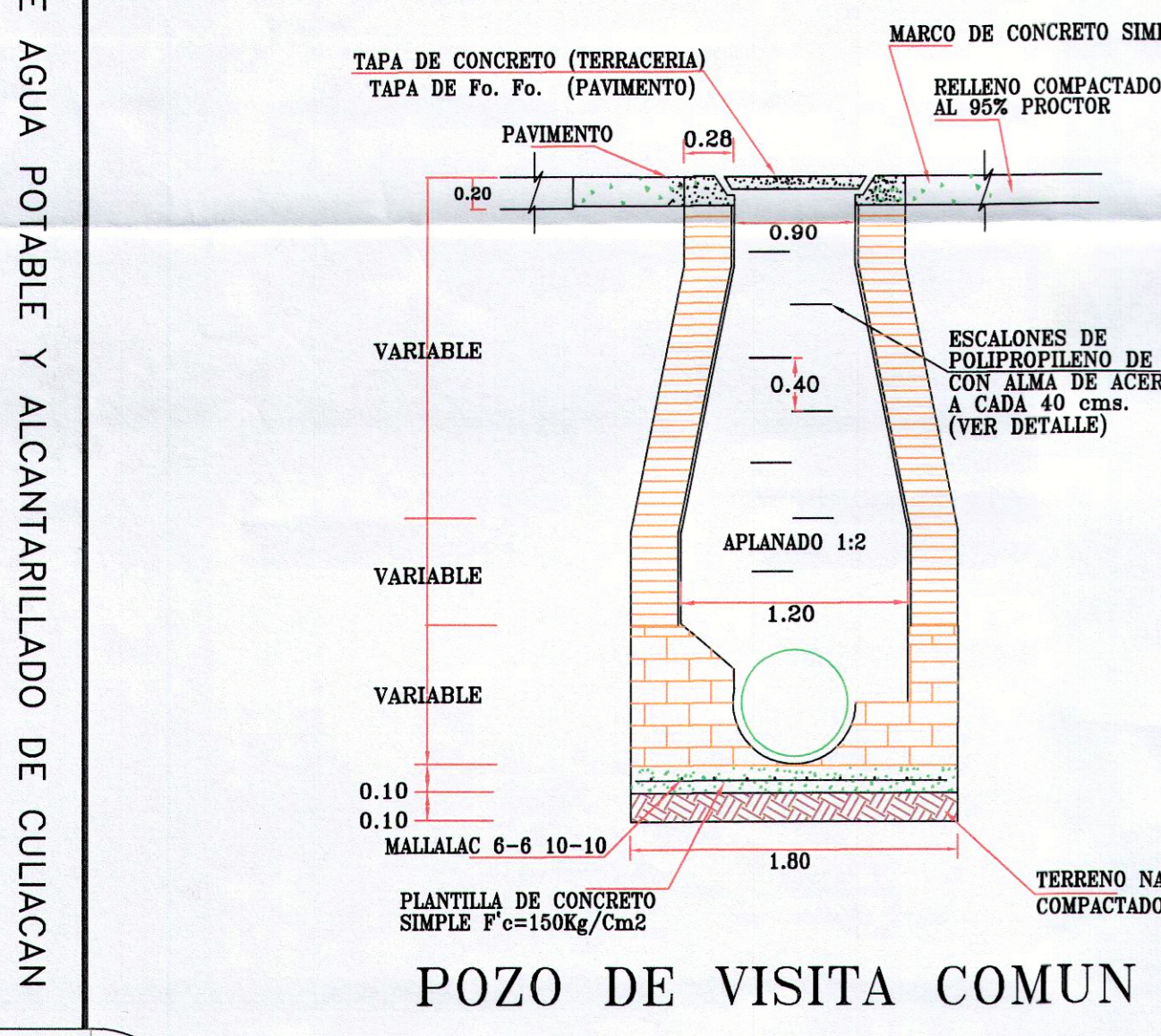
POZO DE VISITA COMUN
