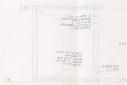
04 CORTE A-A' MODEL SIN ESCALA
