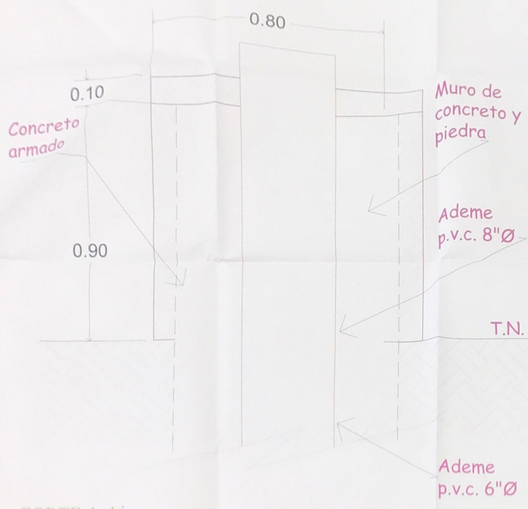
CORTE A-A' FUERA DE ESCALA
