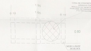
02 PLANTA CIMENTACIÓN MODEL SIN ESCALA
