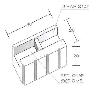
ARQUÍBLOCK CUATRO ESTRIAS ISOMÉTRICO DALA DE CERRAMIENTO TIPO "U" 20X20X40CM. CON 4 ESTRIAS
