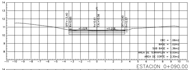
ESTACION 0+090.00
