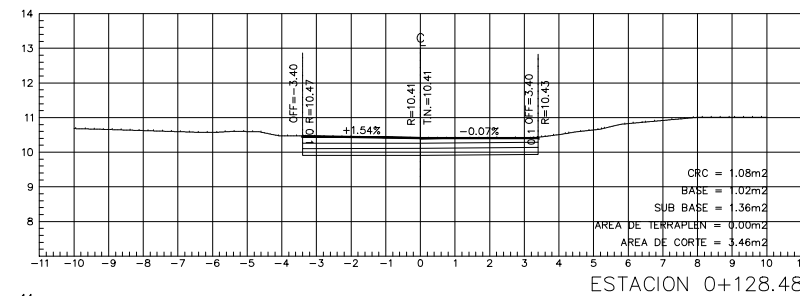
ESTACION 0+128.48
