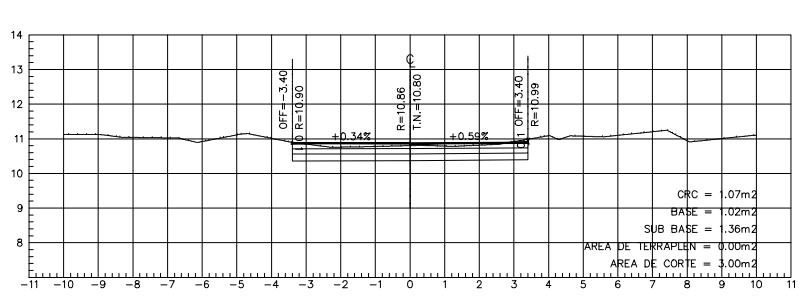
ESTACION 0+040.00
