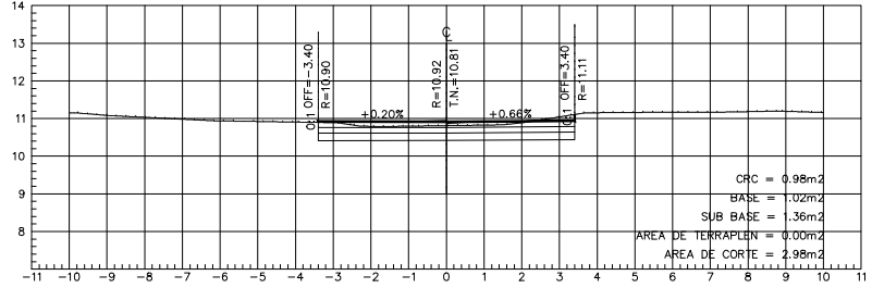
ESTACION 0+030.00
