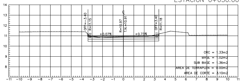
ESTACION 0+020.00
