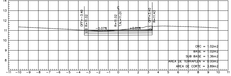
ESTACION 0+010.00
