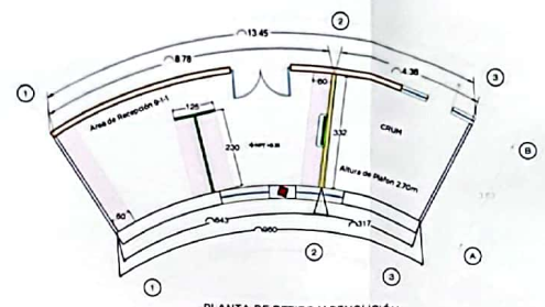
PLANTA DE RETIRO Y DEMOLICIÓN
