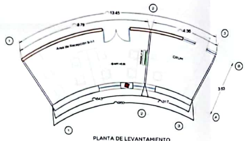
PLANTA DE LEVANTAMIENTO
