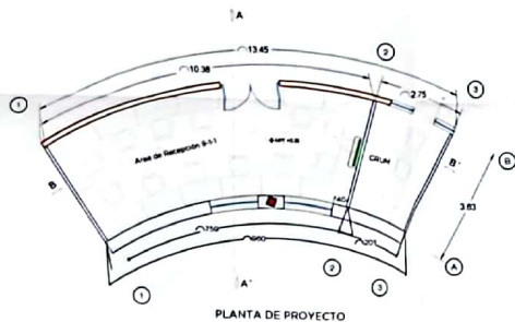
PLANTA DE PROYECTO
