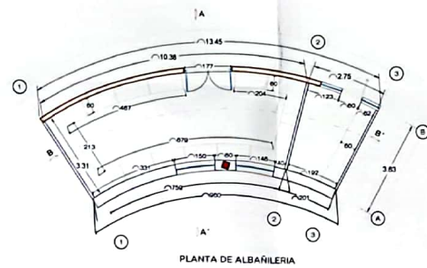
PLANTA DE ALBAÑILERÍA
