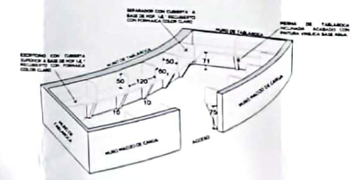
ISOMETRICO AREA 911
