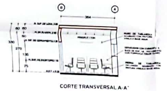
CORTE TRANSVERSAL A-A'
