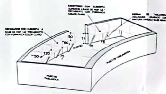
ISOMETRICO AREA 911
