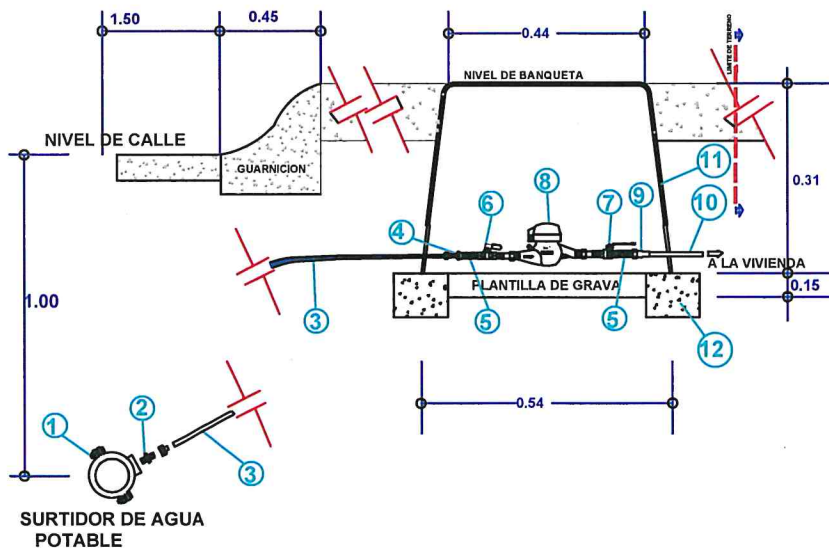
DETALLE DE MEDIDOR Y COMPONENTES CON CAJA DE POLIETILENO.
