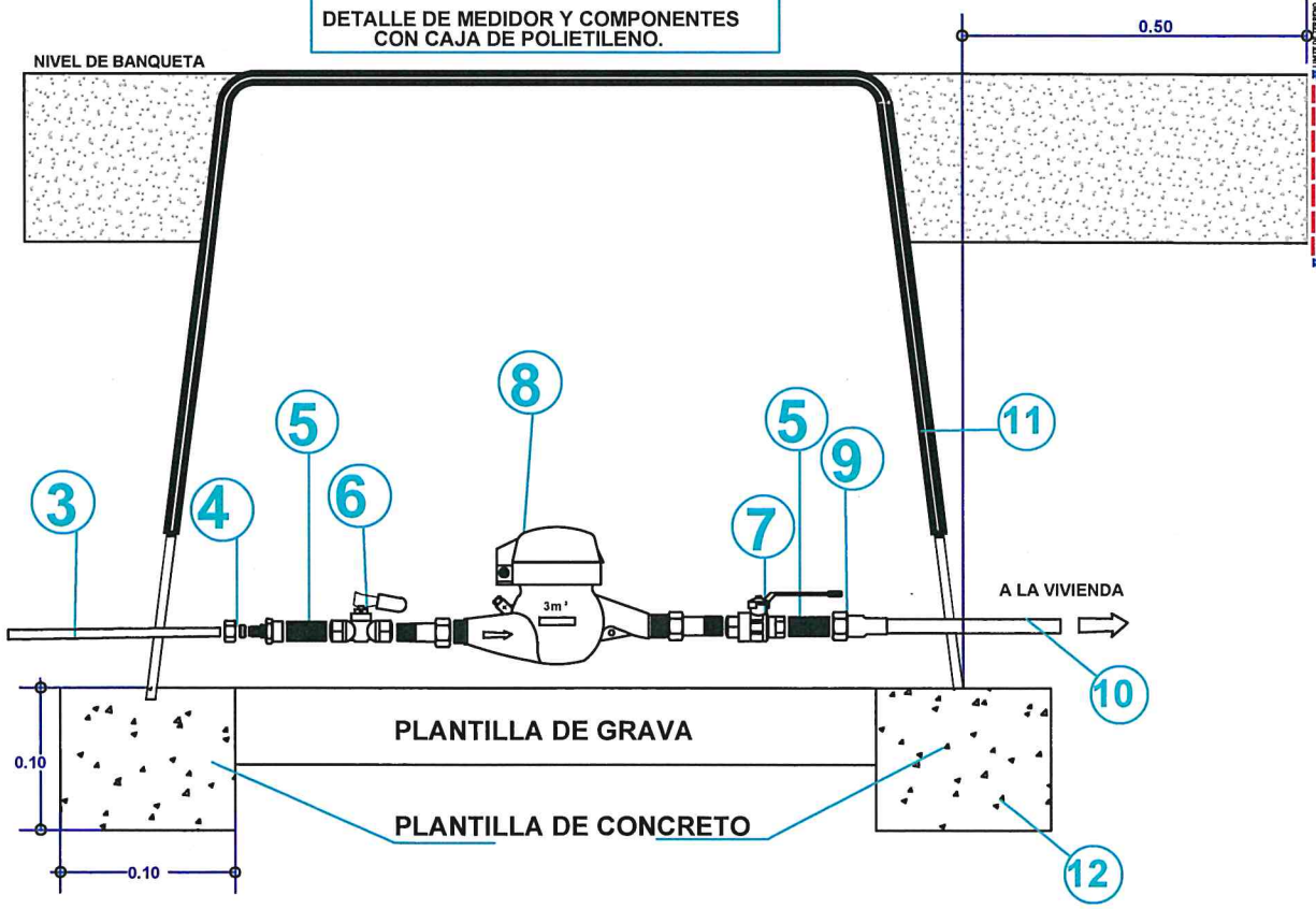
TOMA DOMICILIARIA CON CAJA DE MEDICION DE POLIETILENO
