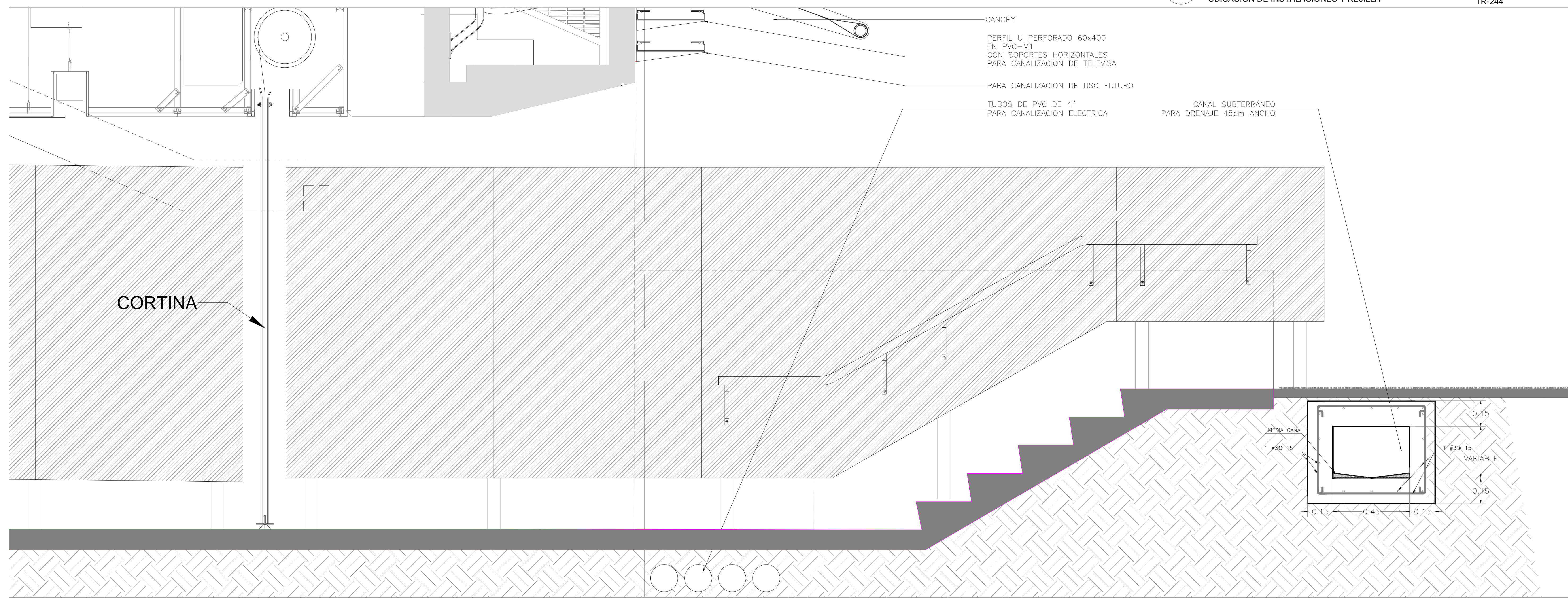
02 SECCION A NIVEL DE CANCHA 1:25 UBICACION DE INSTALACIONES EN TUNEL DE JUGADORES TR-244
