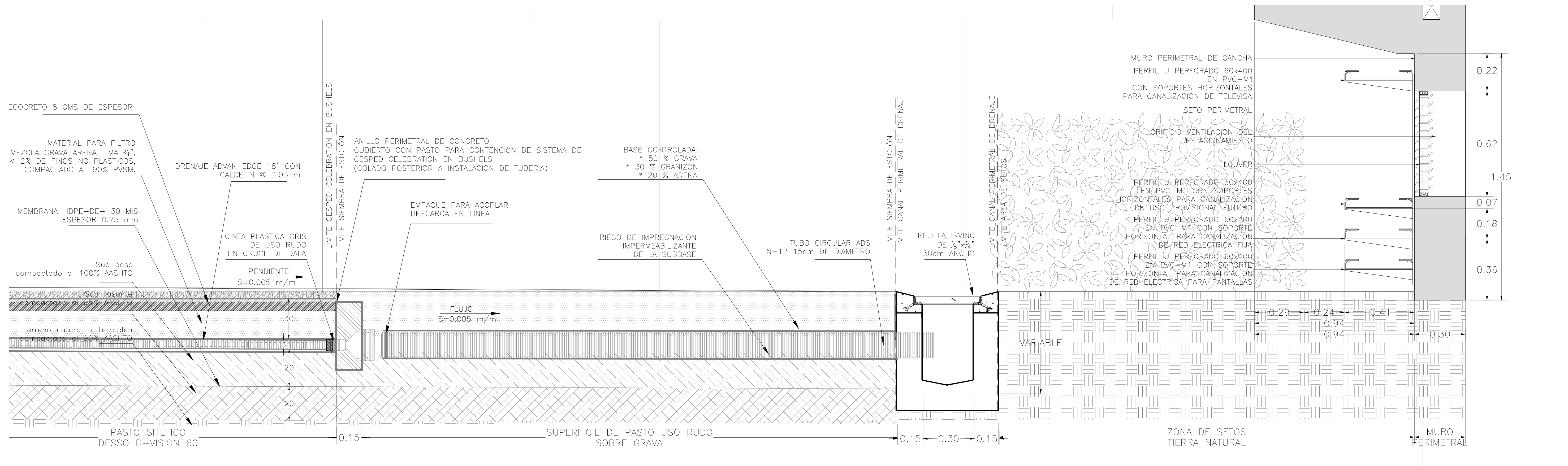
01 SECCION A NIVEL DE CANCHA 1:25 UBICACION DE INSTALACIONES Y REJILLA TR-244
