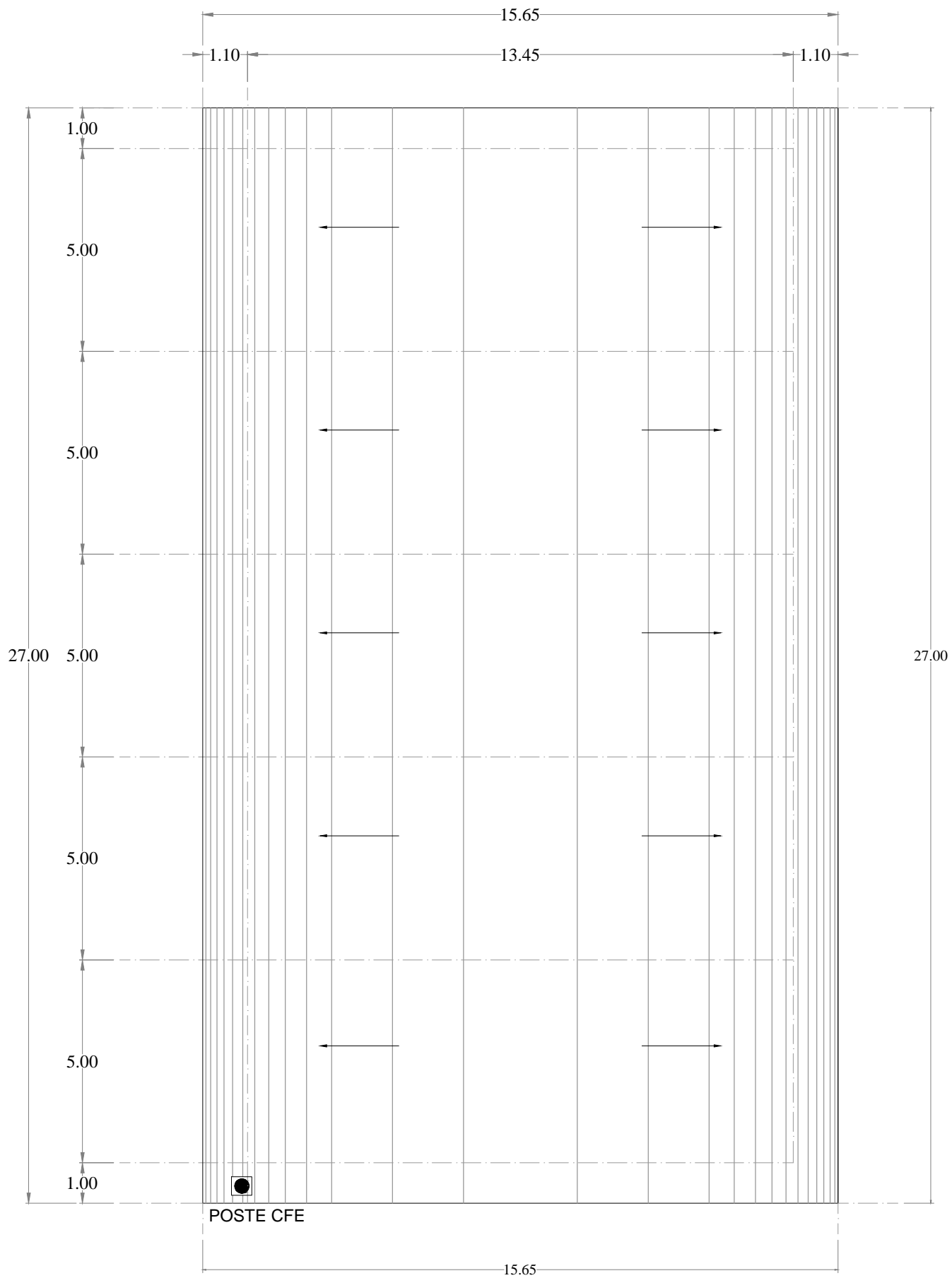
PLANTA DE AZOTEA
