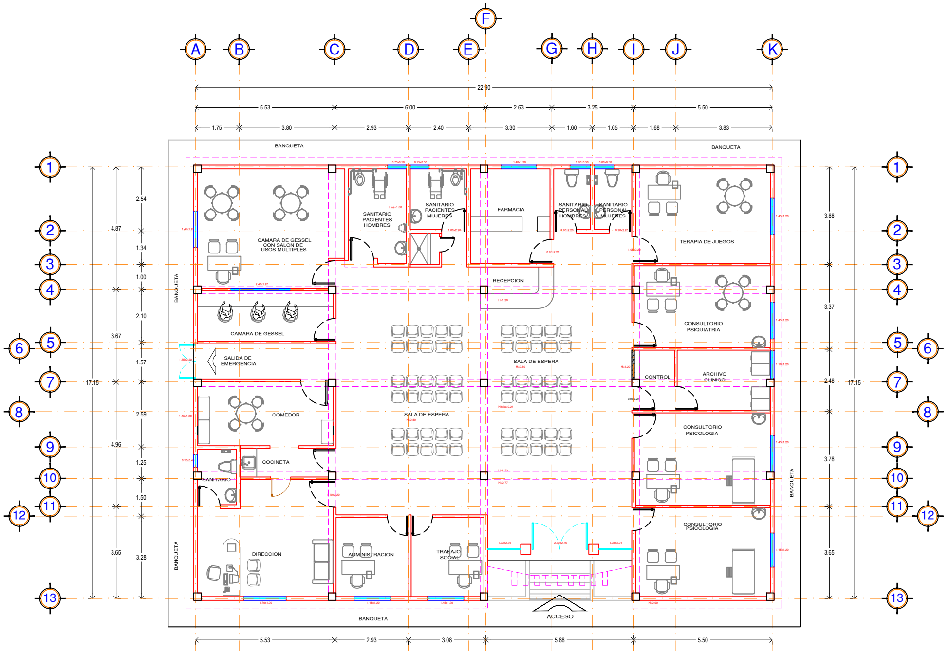
PLANTA ARQUITECTONICA UNEME CISAME (Salud MEntal) CULIACAN
