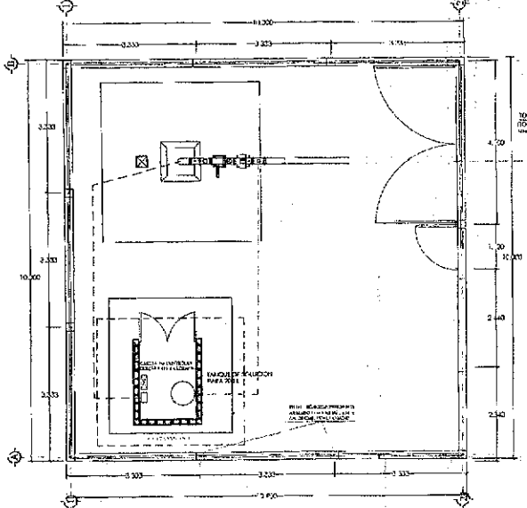
PLANTA DE CERCA Y SEMBRADO DE PILOTES EN POZO ESC. 1:50.
