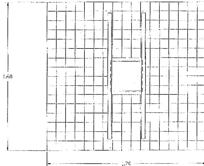
TIPO 3 MURUS DE TABIQUE 28 cms.
