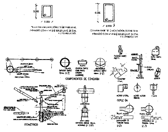
SECCION DE CERCA ACCESO EN POZO ESC. 1:20.
