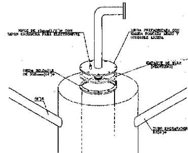
DETALLE DE SOPORTE DE ARREGLOS HIDRAULICOS
