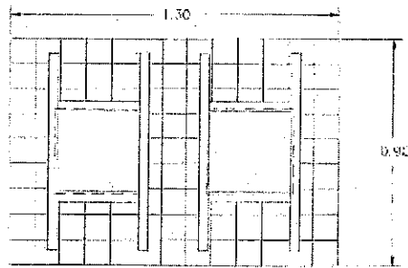
TIPO 5 MUROS DE TABIQUE 14 CM.
