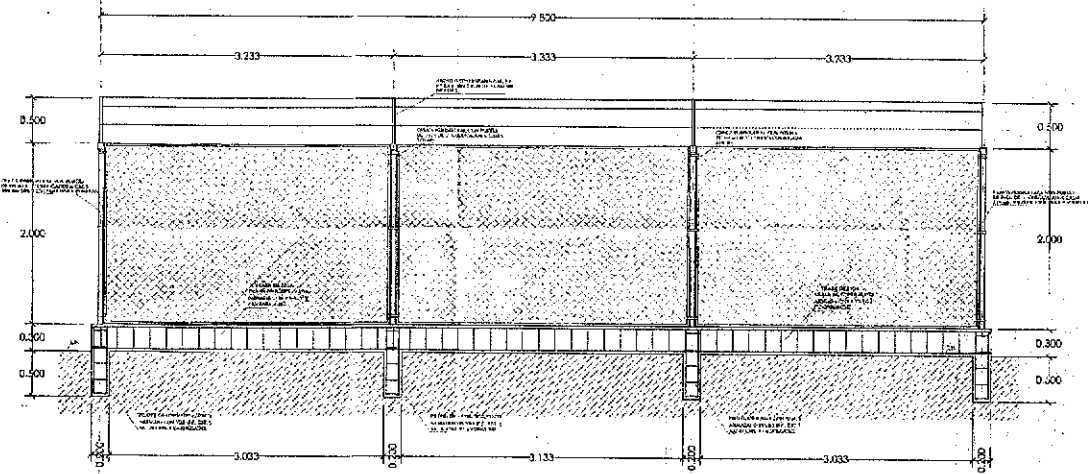
SECCION LATERAL DE CERCA EN POZO ESC. 1:20.
