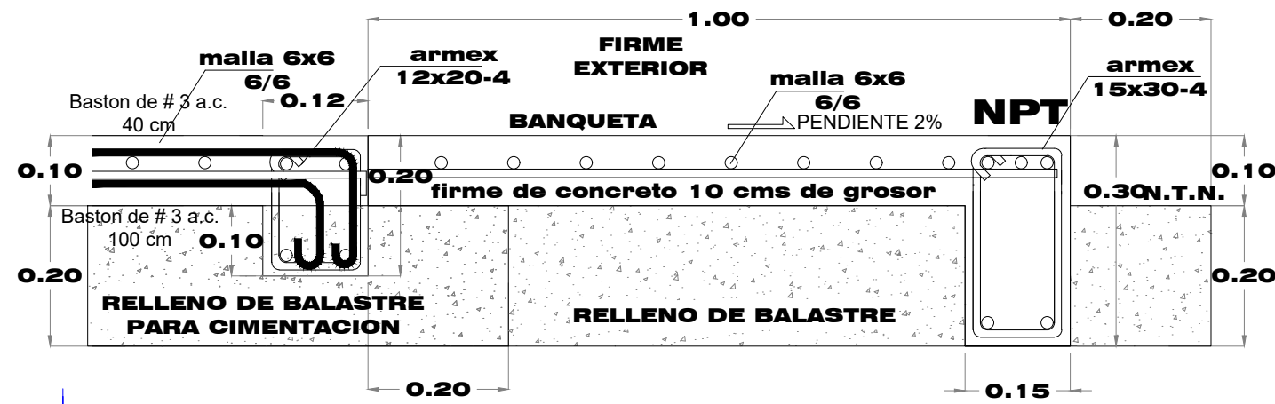
DETALLE DE FIRME DE CONCRETO EN ACCESO
