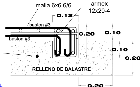
DETALLE DE CIMENTACION CORTE A-A'
