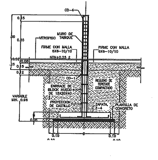
CORTE E-E
