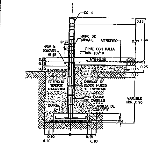
CORTE B-B
