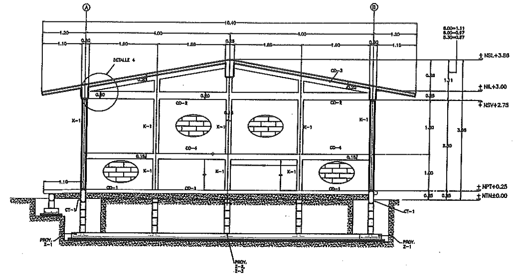
CORTE ESTRUCTURAL TRANSVERSAL
