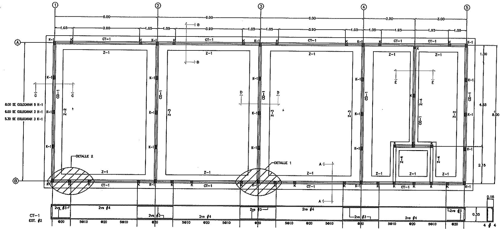
PLANTA DE CIMENTACIÓN (AGRUPAMIENTO MAXIMO 4 AULAS)
