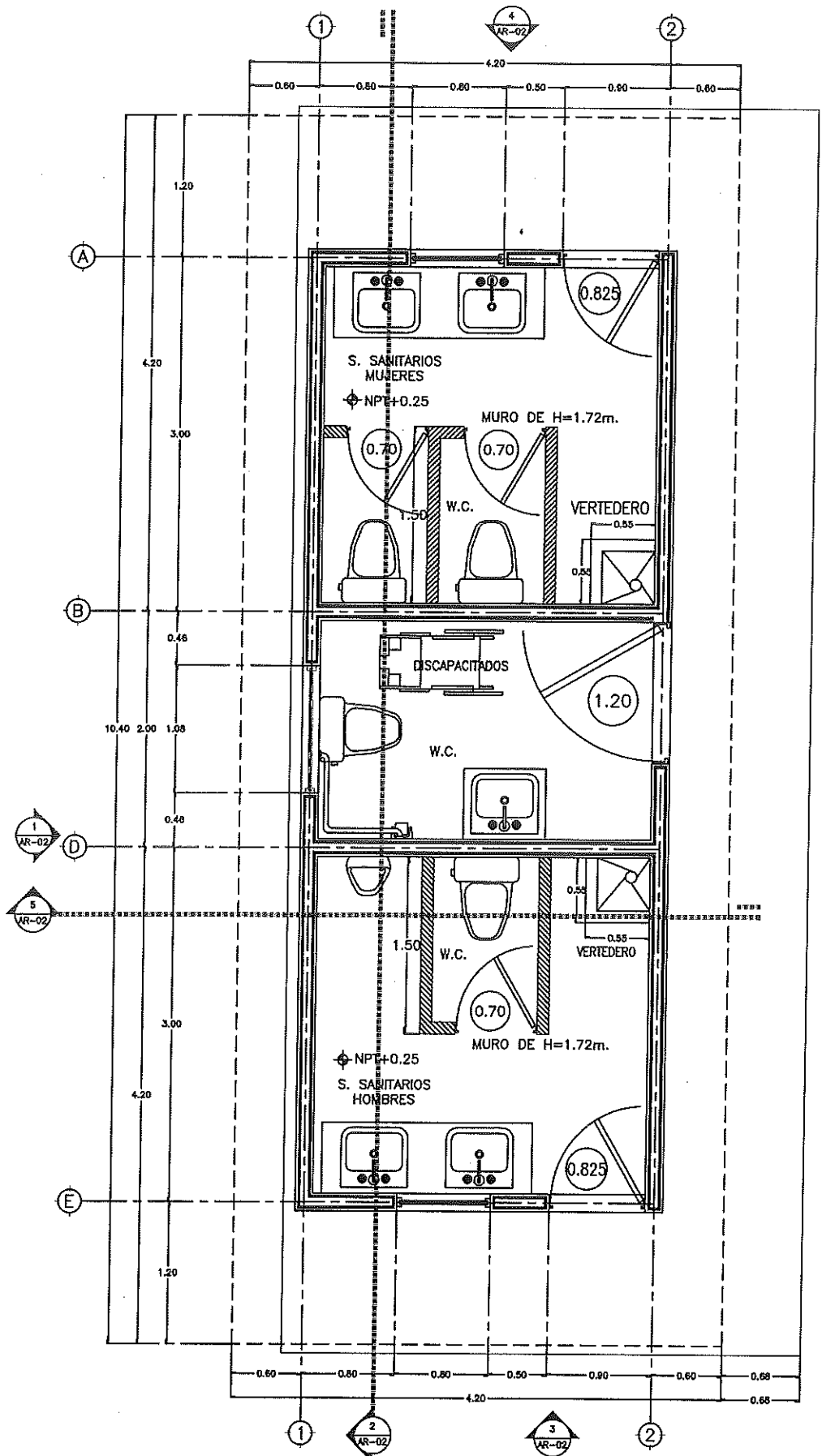
1 PLANTA ARQUITECTONICA
