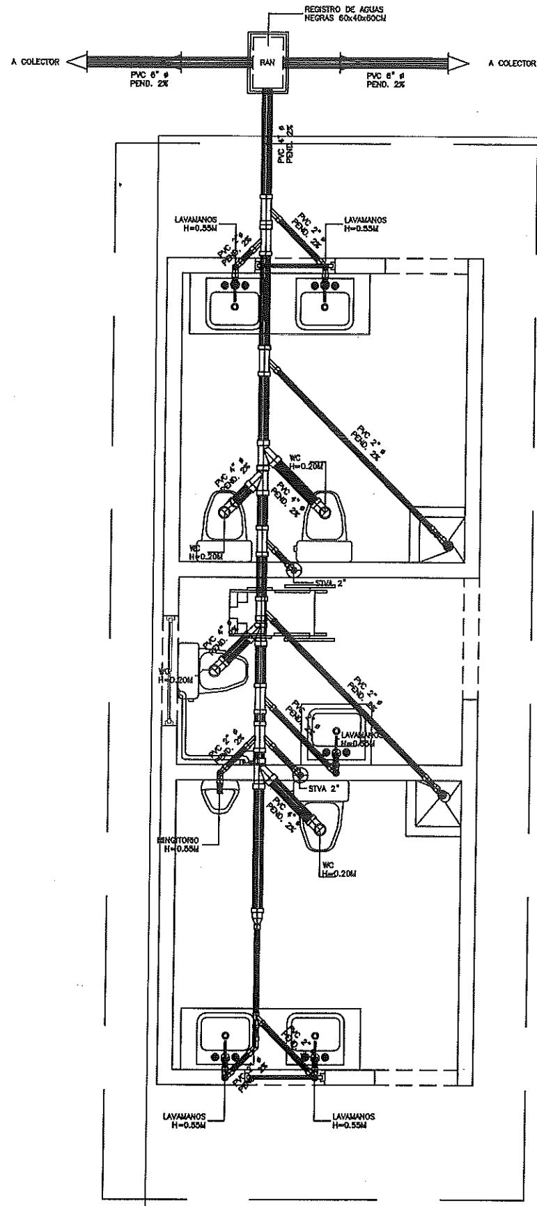
1 PLANTA INSTALACIÓN SANITARIA ESC, 1:50
