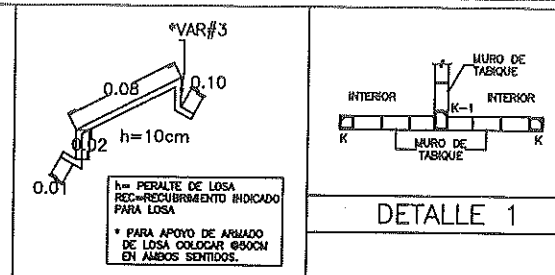
DETALLE DE SILLETA
