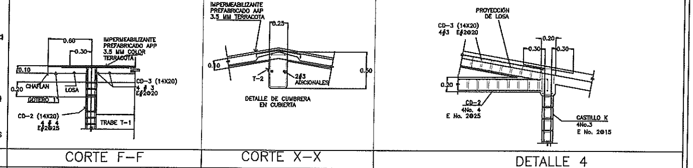
CORTE ESTRUCTURAL TRANSVERSAL
