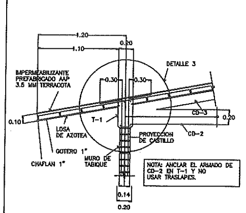
CORTE E-E
