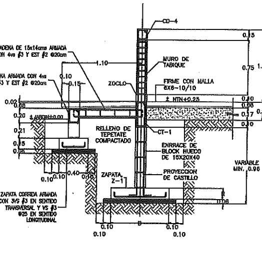
CORTE A-A
