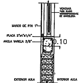
DETALLE DE HERRERIA
