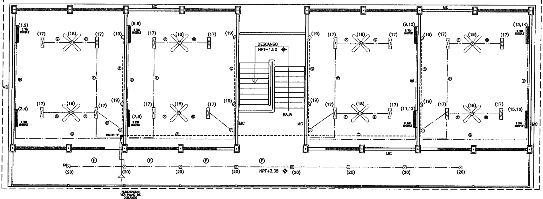
INSTALACION ELECTRICA - PLANTA ALTA
