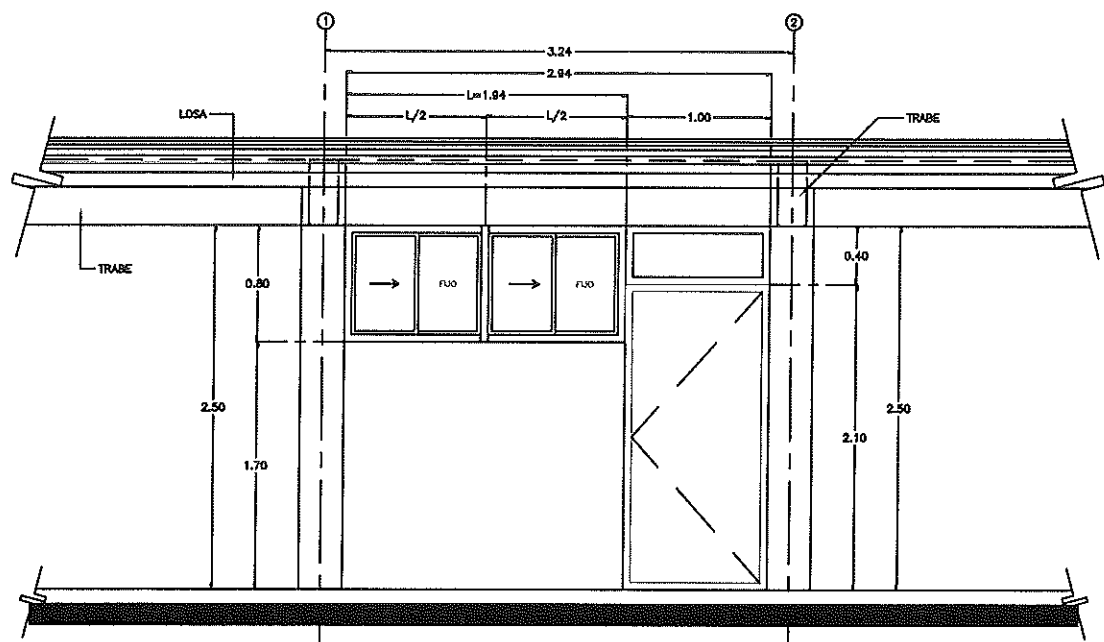
1 CANCELERIA EN FACHADA PRINCIPAL - MUROS BAJOS
