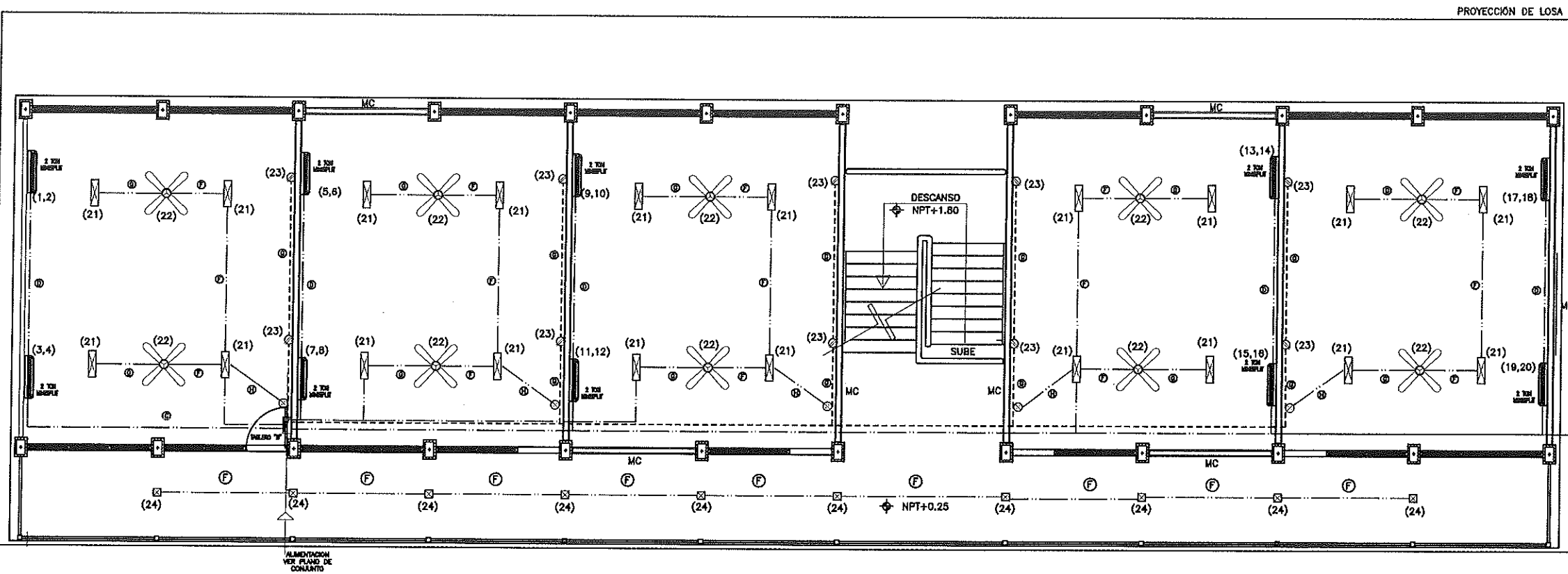
INSTALACION ELECTRICA - PLANTA ALTA
