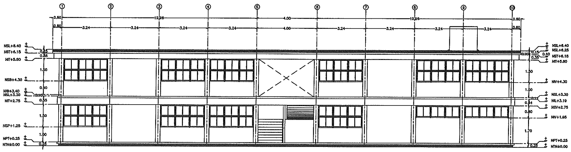
2 FACHADA POSTERIOR ESC. 1:75
