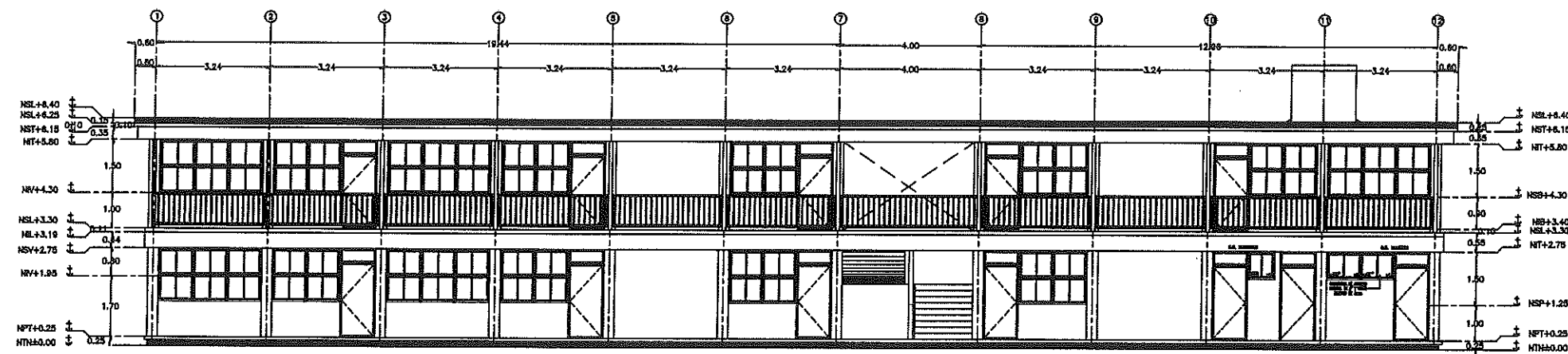
1 FACHADA FRONTAL ESC. 1:75
