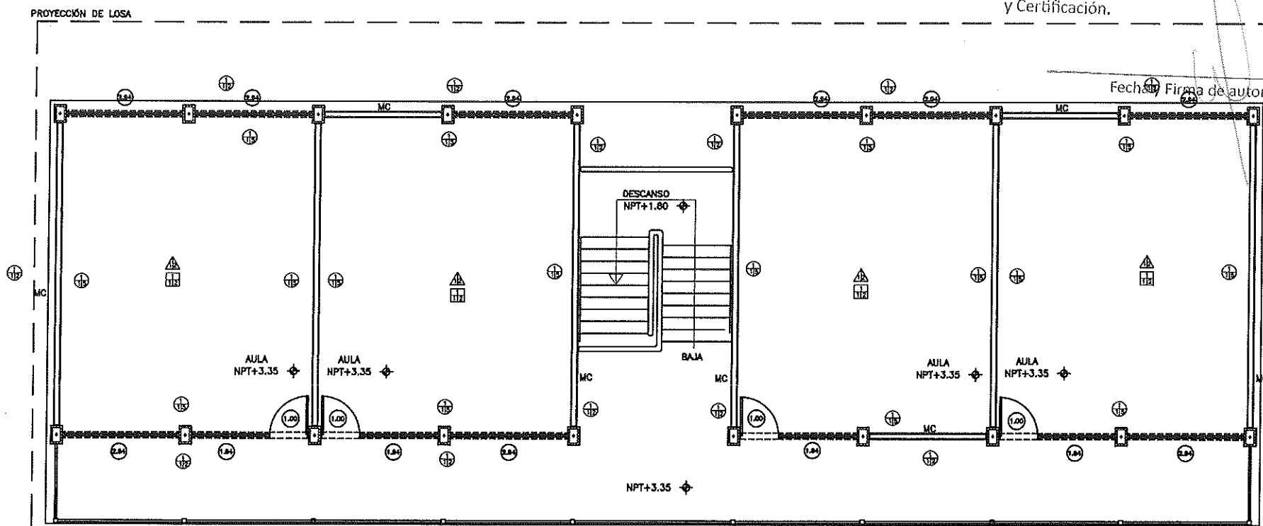
2 PLANTA ARQUITECTONICA ALTA
