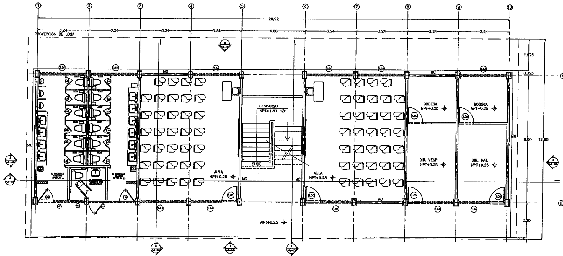
1 PLANTA ARQUITECTONICA BAJA
