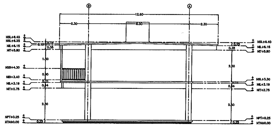
4 FACHADA LATERAL ESC. 1:75
