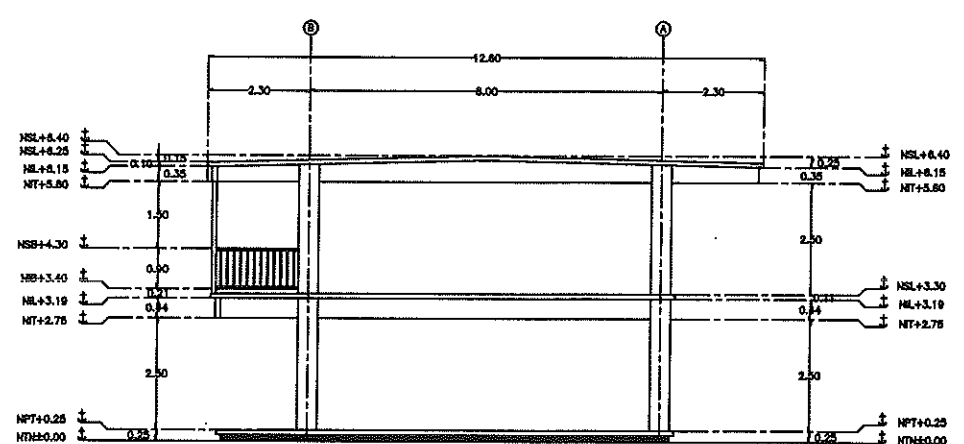
2 FACHADA POSTERIOR ESC. 1:75
