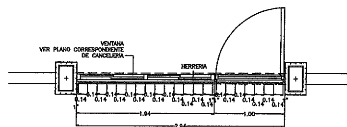
HERRERIA EN FACHADA PRINCIPAL – AULAS
