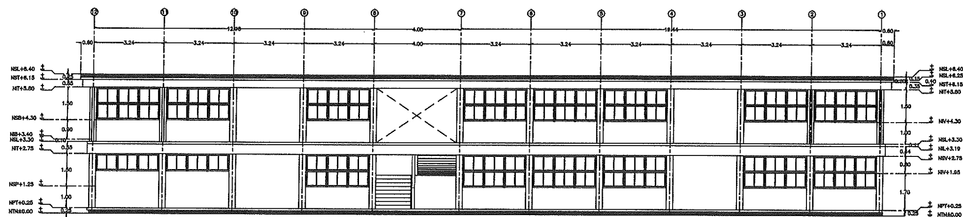
2 FACHADA POSTERIOR ESC. 1:75
