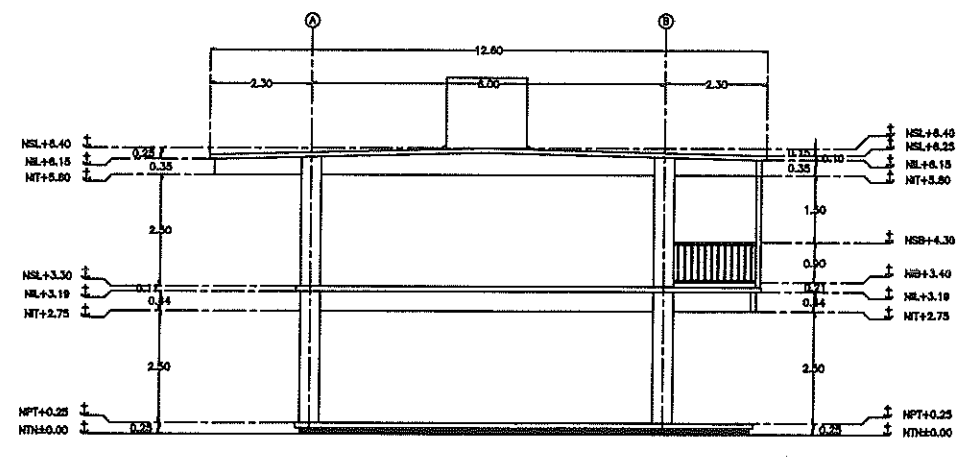
3 FACHADA LATERAL ESC. 1:75
