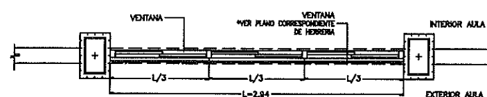
4 CANCELERIA EN FACHADA POSTERIOR - MUROS ALTOS
