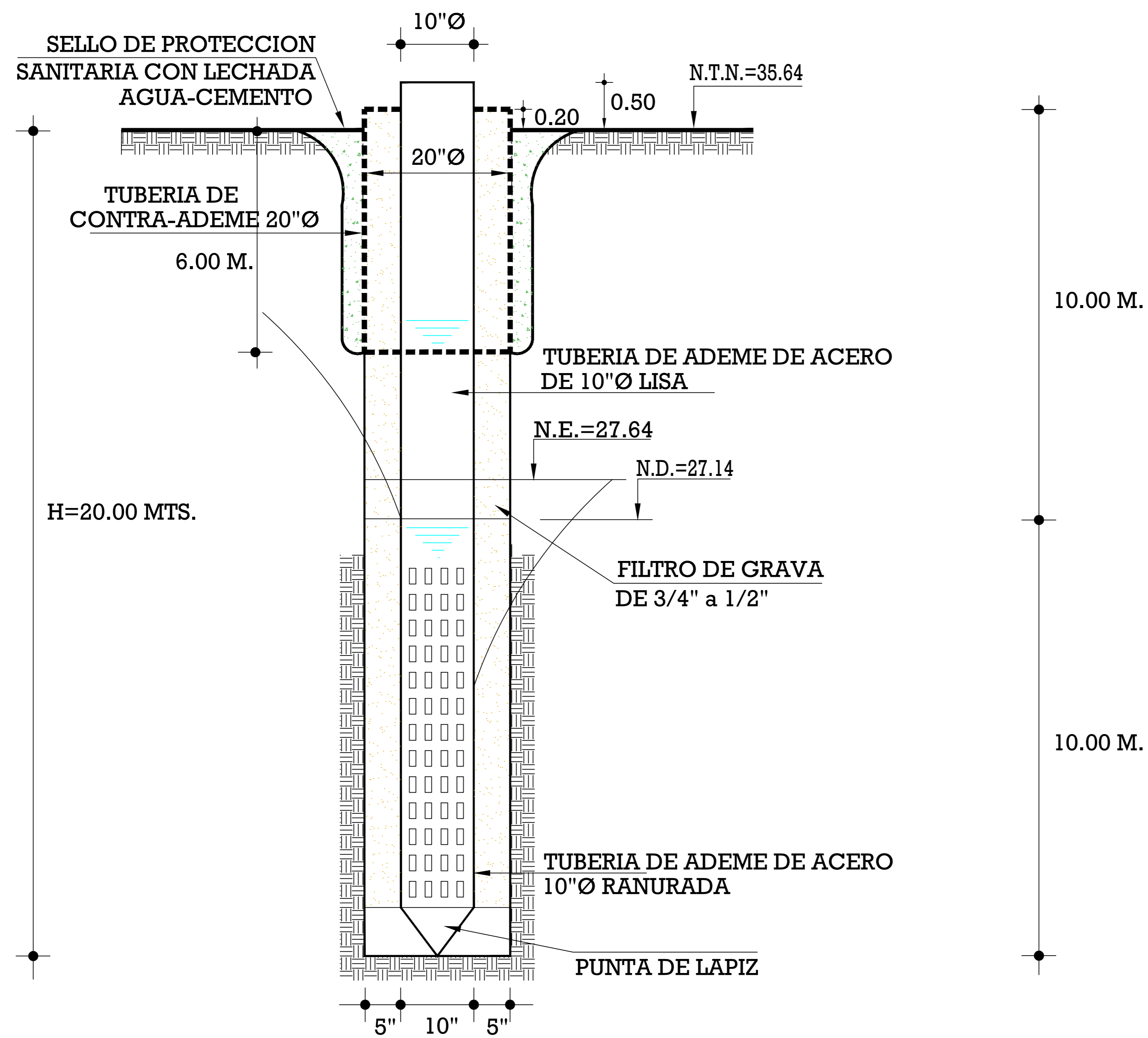
DETALLE DE POZO TIPO PROFUNDO S/E
