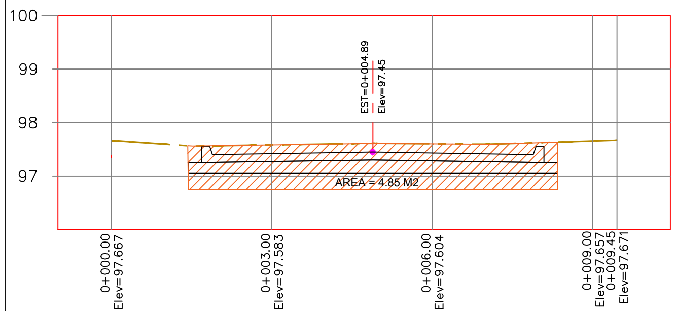
PERFIL 0+120
