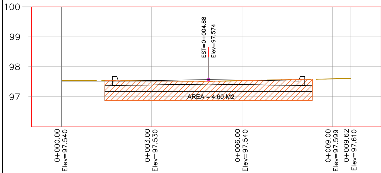
PERFIL 0+100
