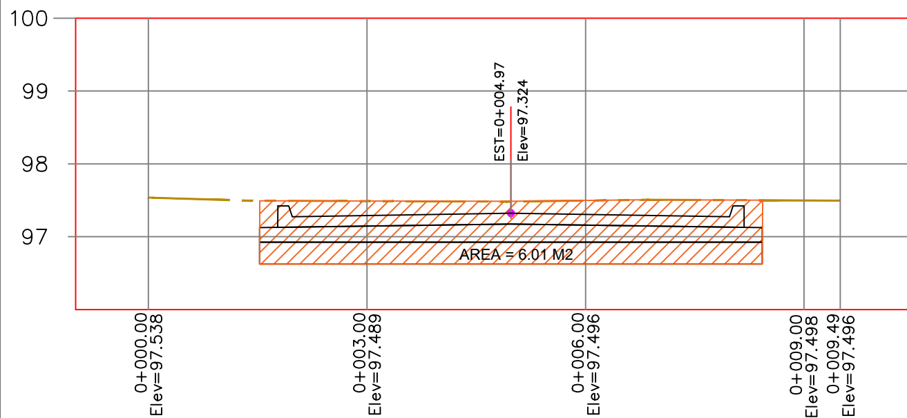
PERFIL 0+140
