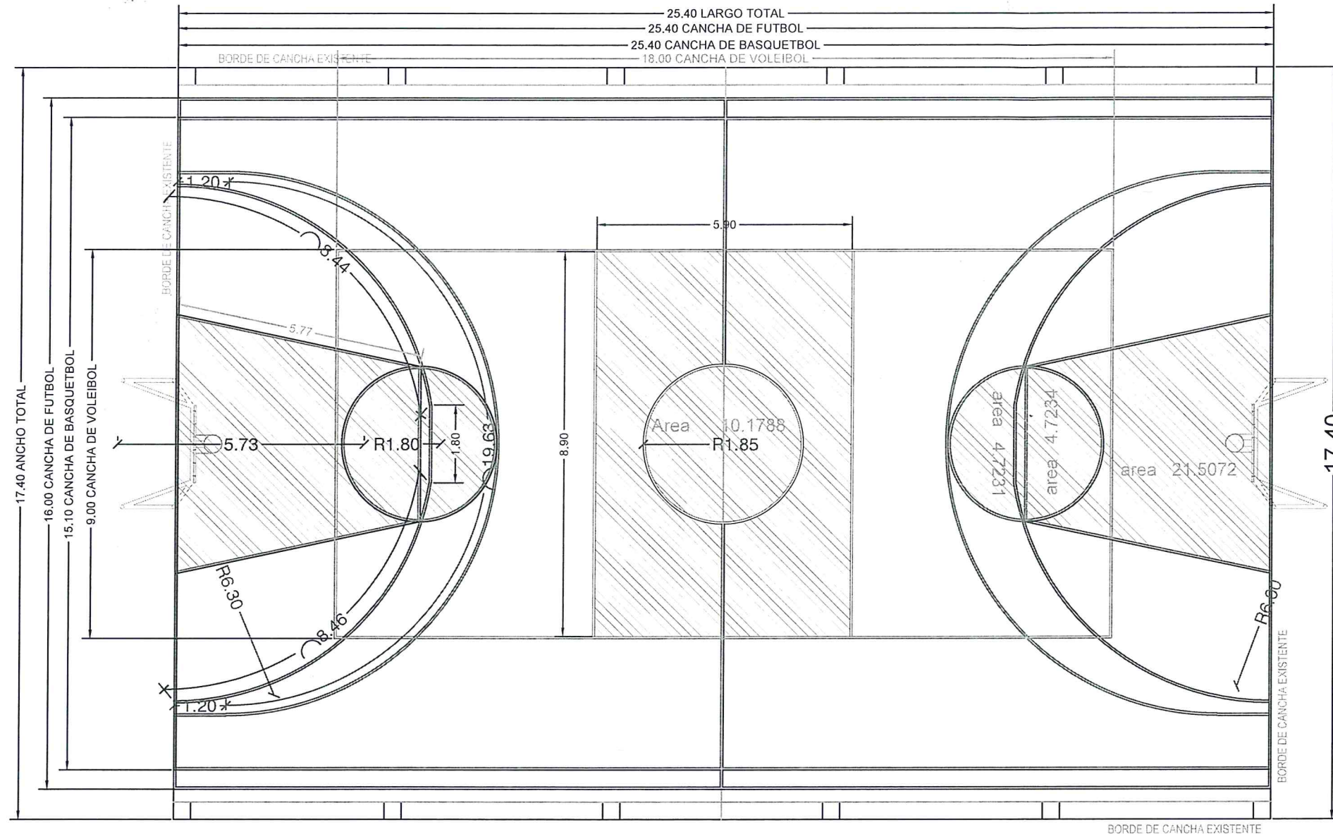
1 PLANTA DE CONJUNTO SIN ESCALA
