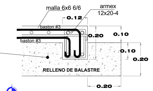
DETALLE DE CIMENTACION CORTE A-A'
