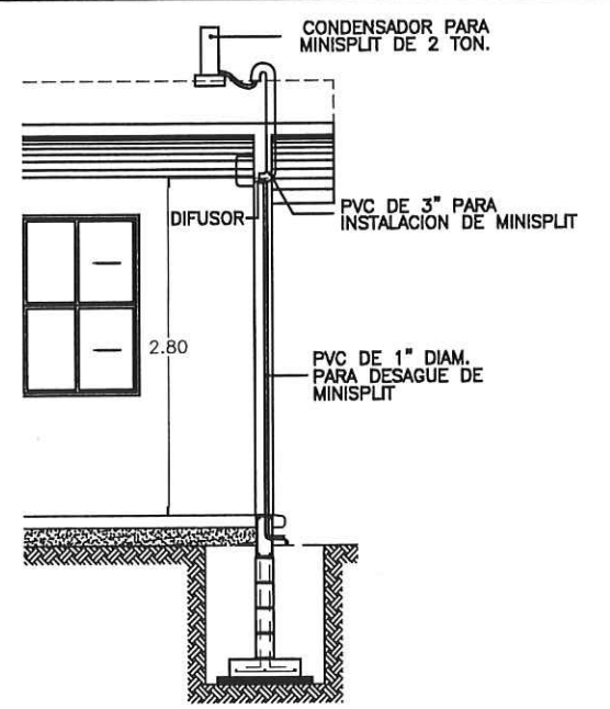
2 DETALLE DE MINI-SPLIT S / E
