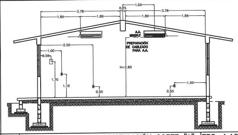
4 DET. DE ALTURAS EN INSTALACIÓN CORTE "A" ESC. 1:100
