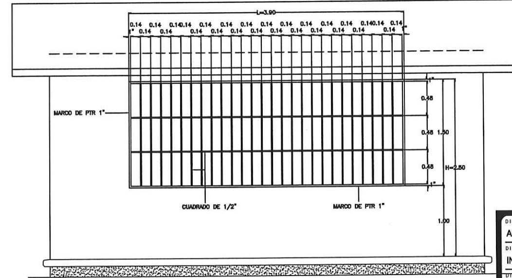
2 HERRERIA EN FACHADA PRINCIPAL – AULAS ESC. 1:50
