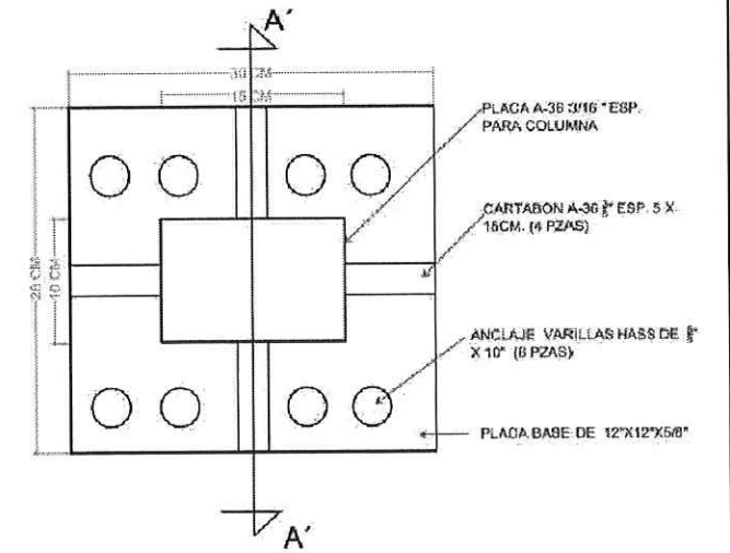
DETALLE ANCLAJE COL-DADO
