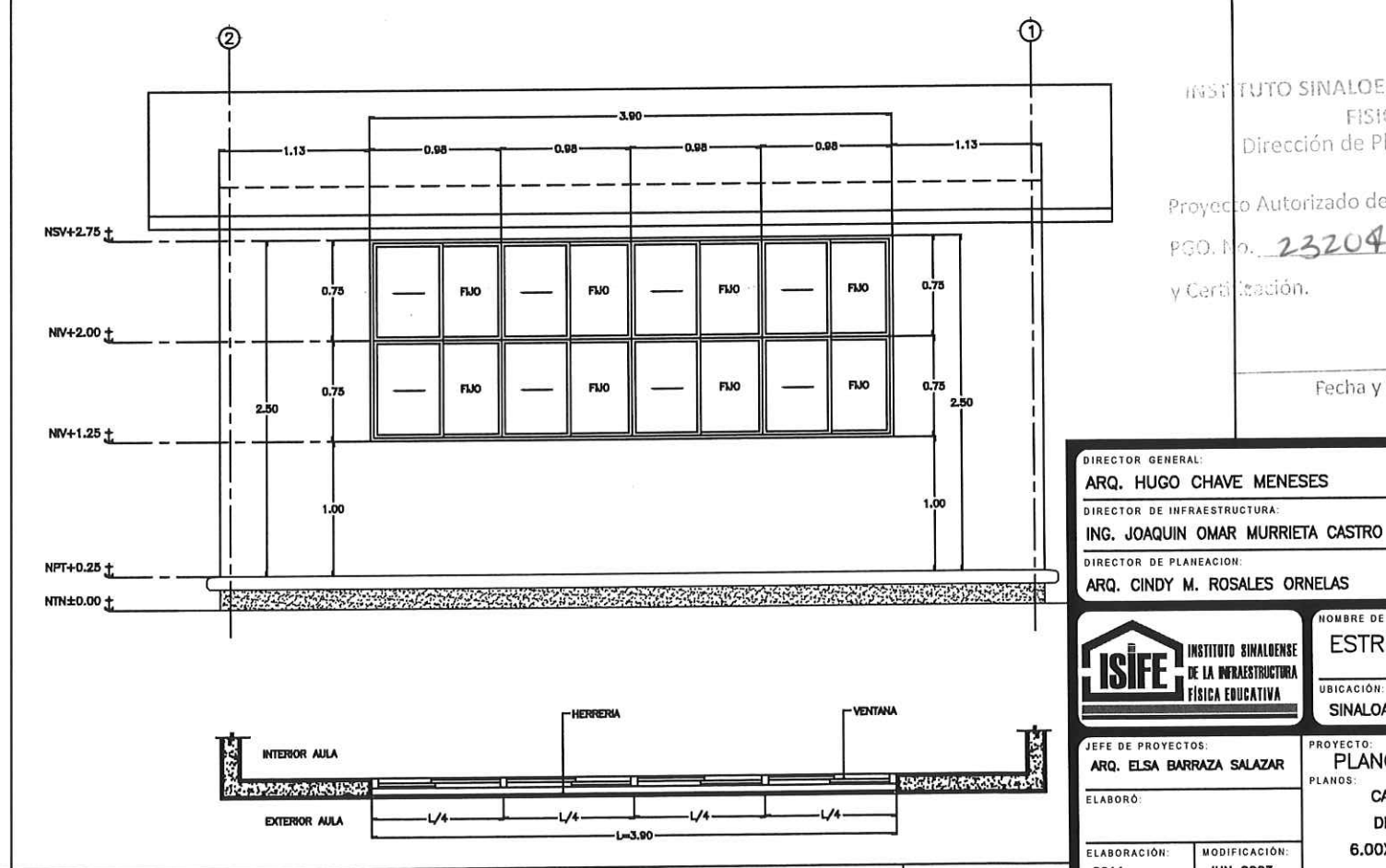
4 CANCELERIA EN FACHADA POSTERIOR - AULAS ESC. 1:50
