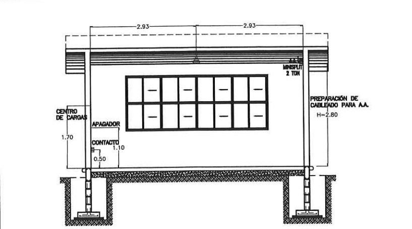
5 DETALLE DE ALTURAS EN INSTALACIÓN CORTE "B" ESC. 1:100
