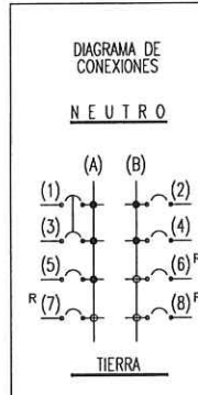
2 CABLEADO S / E
