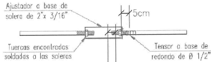
DETALLE "A"
