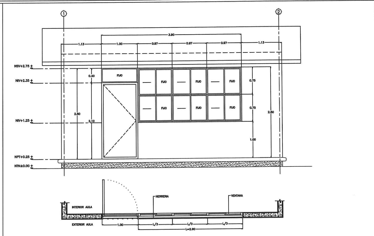
2 CANCELERIA EN FACHADA PRINCIPAL-AULAS ESC. 1:50
