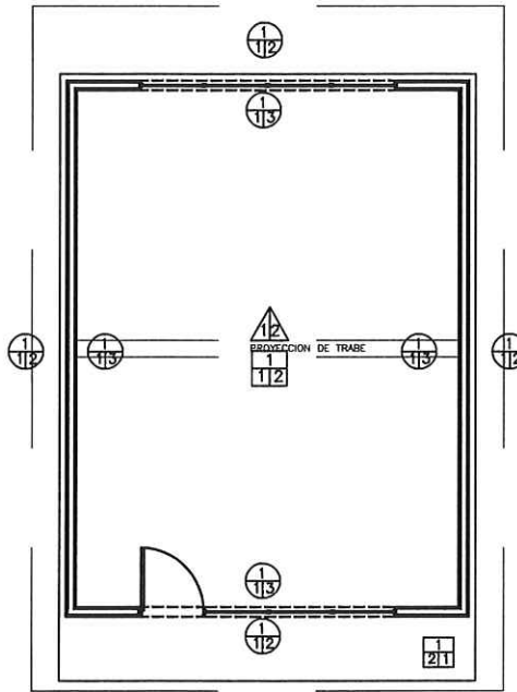
4 ACABADOS EN PLANTA ARQUITECTÓNICA
