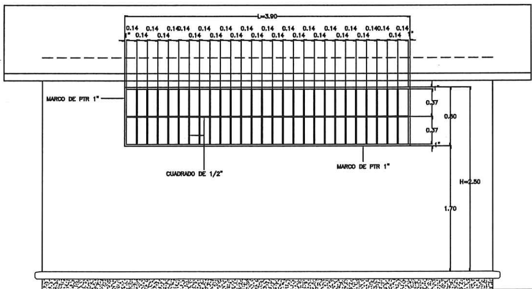
1 HERRERIA EN FACHADA PRINCIPAL – TALLERES Y LABORATORIOS ESC. 1:50
