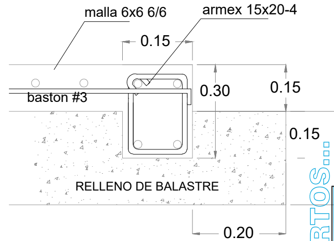
Detalle de cimentacion corte A-A'
