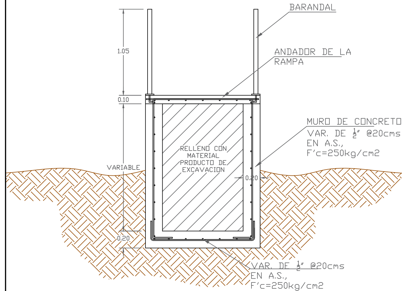
DETALLE DE RAMPA.-
