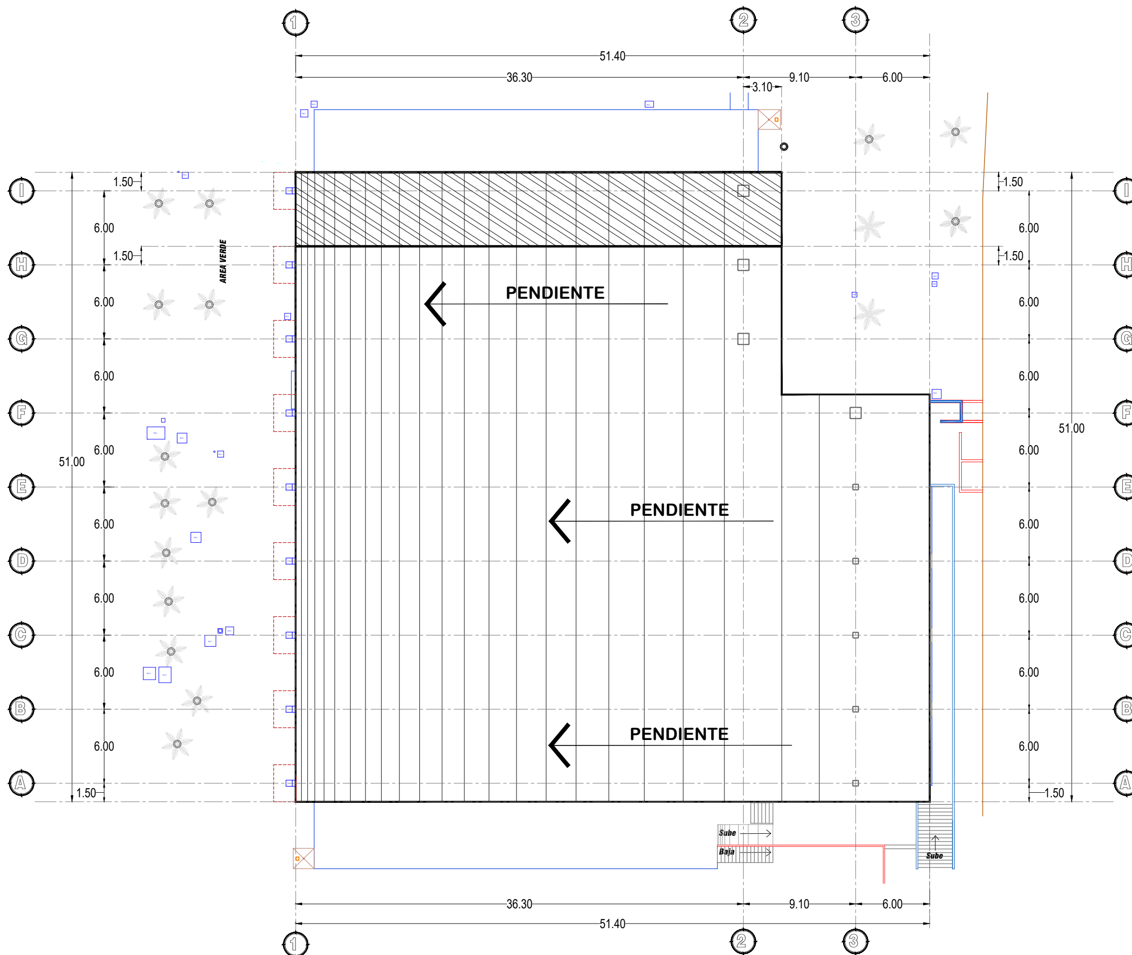
PLANTA ARQUITECTÓNICA DE AZOTEA
