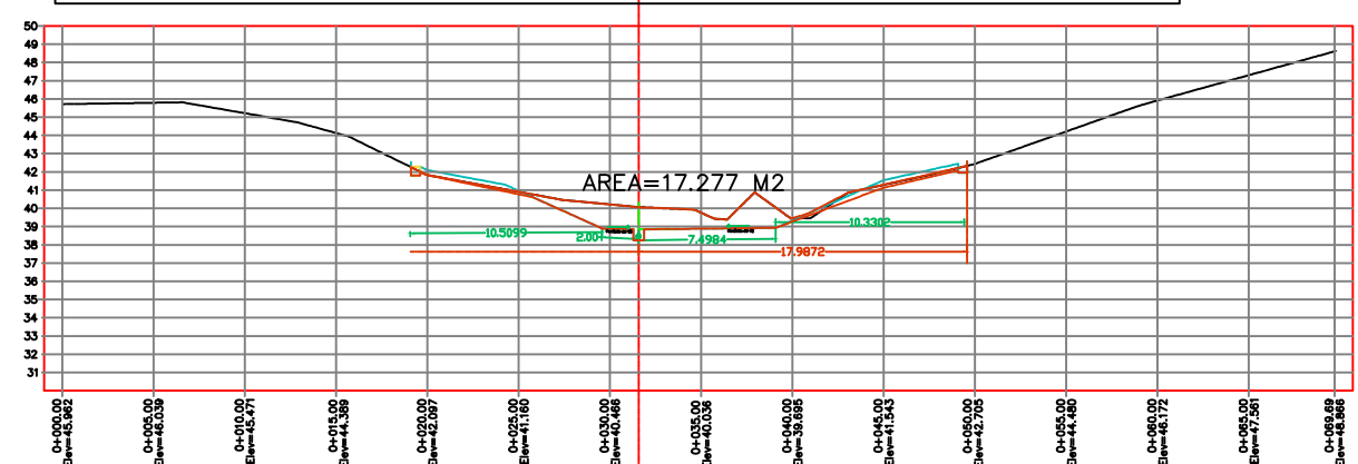
PERFIL 0+227 ESCALA HORIZONTAL 1 : 100 ESCALA VERTICAL 1 : 100 VOLUMEN DE CORTE=381.60 M3
