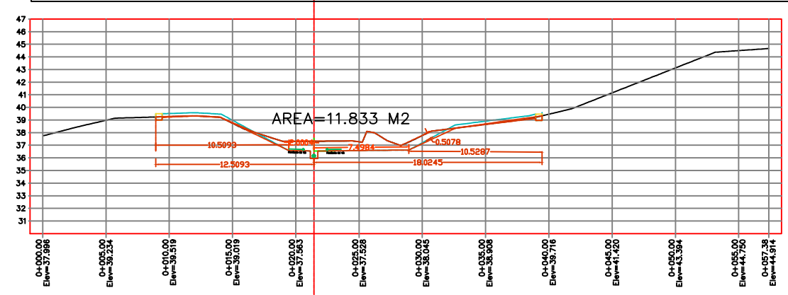
PERFIL 0+267 ESCALA HORIZONTAL 1 : 100 ESCALA VERTICAL 1 : 100 VOLUMEN DE CORTE=138.40 M3
