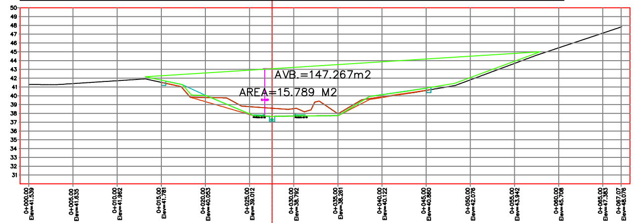
PERFIL 0+267 ESCALA HORIZONTAL 1 : 100 ESCALA VERTICAL 1 : 100 VOLUMEN DE CORTE=138.40 M3
