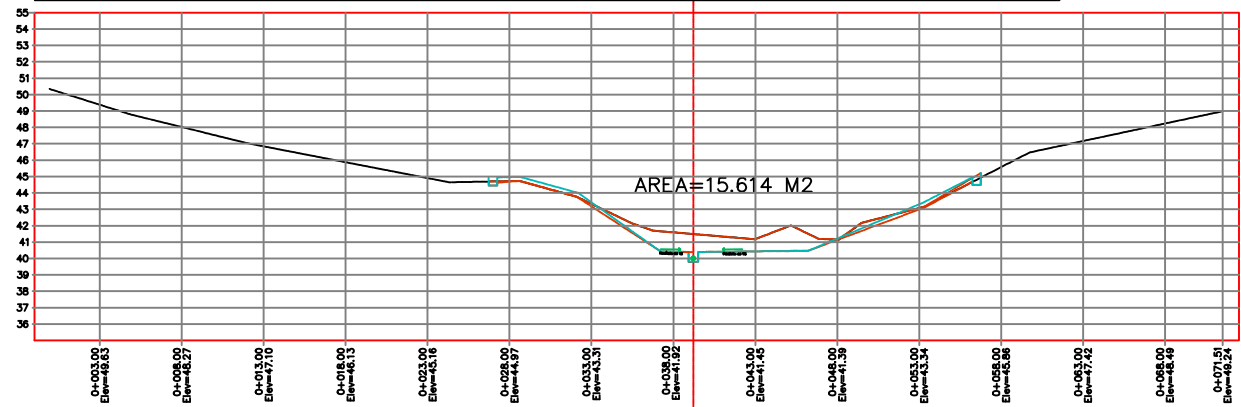
PERFIL 0+207 ESCALA HORIZONTAL 1 : 100 ESCALA VERTICAL 1 : 100 VOLUMEN DE CORTE=377.80 M3
