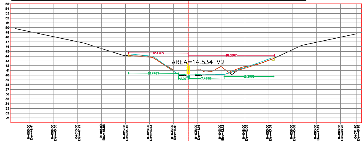
PERFIL 0+207 ESCALA HORIZONTAL 1 : 100 ESCALA VERTICAL 1 : 100 VOLUMEN DE CORTE=377.80 M3
