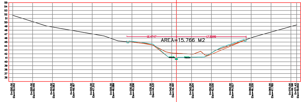
PERFIL 0+167 ESCALA HORIZONTAL 1 : 100 ESCALA VERTICAL 1 : 100 VOLUMEN DE CORTE=349.15 M3
