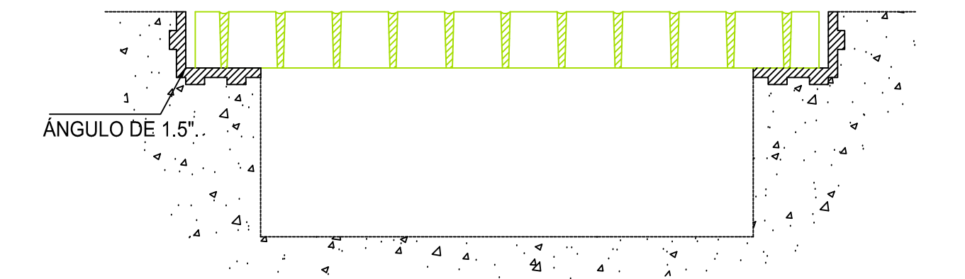
REJILLA MOLDEADA RECTANGULAR SUPERIOR PARA AREA DE MANTENIMIENTO PEATONAL CON MATERIAL DE RESINA DE POLIESTER TIPO ROVING AL 70% DE RESINA DE PESO TIPO ANTIDERRAPANTE 4'x12' CON PERALTE DE 1.5" PARA CUBRIR UN AREA DE 4.0 M2 INCLUYE: 3 ÁNGULOS DE 1.5".
