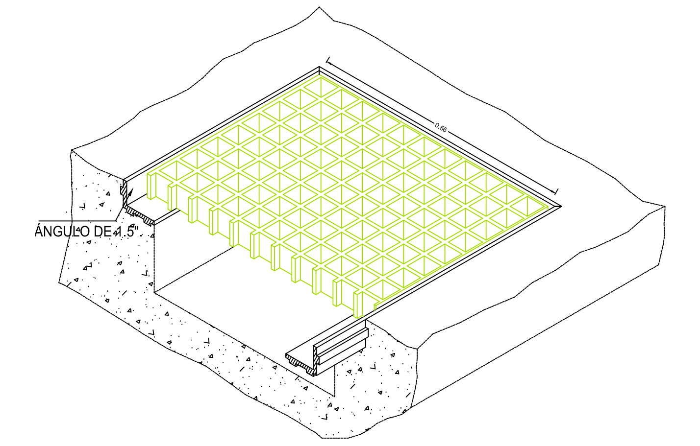
REJILLA MOLDEADA RECTANGULAR SUPERIOR PARA AREA DE MANTENIMIENTO PEATONAL CON MATERIAL DE RESINA DE POLIESTER TIPO ROVING AL 70% DE RESINA DE PESO TIPO ANTIDERRAPANTE 4'x12' CON PERALTE DE 1.5" PARA CUBRIR UN AREA DE 4.0 M2 INCLUYE: 3 ÁNGULOS DE 1.5".
