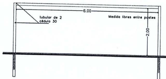
Alzado frontal
