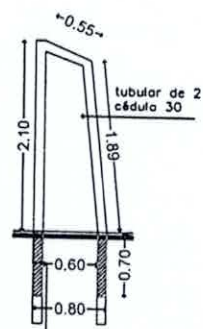
Alzado lateral
