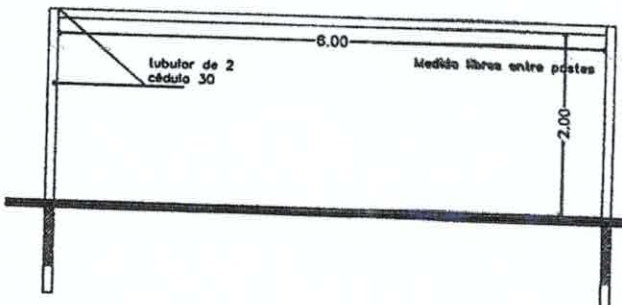
Alzado frontal
