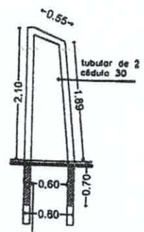
Alzado lateral
