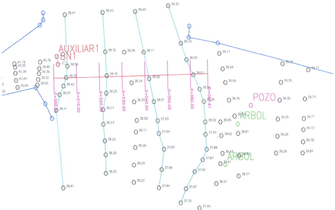
PLANTA TOPOGRAFICA
