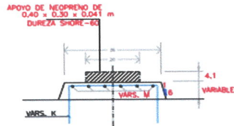
ALZADO TIPO ESCALA 1:20
