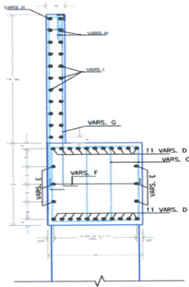
PTE_TYL_2020 ARMADO DE CABEZAL ESCALA 1:20 CONCRETO f_c=250 \text{ kg/cm}^2 ACERO DE REFUERZO f_y=4200 \text{ kg/cm}^2
