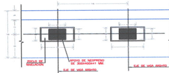
PTE_TYL_2020 DETALLE 1 ESCALA 1:20 DIMENSIONES EN CENTÍMETROS NEOPRENO DUREZA SHORE-60 f_y=100 \text{ kg/cm}^2
