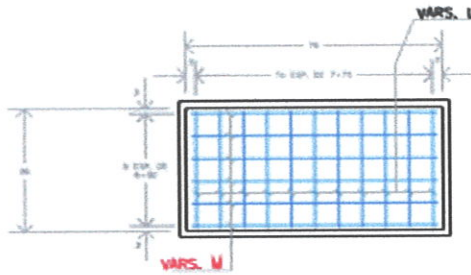
ARMADO ESCALA 1:20
