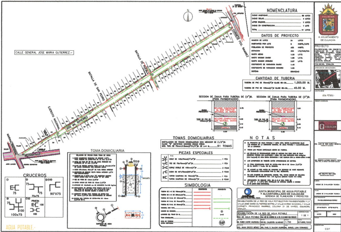
Plano de Agua Potable
