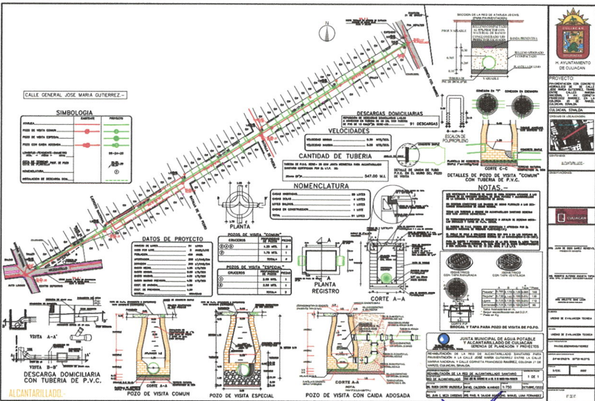
Plano de Drenaje Sanitario
