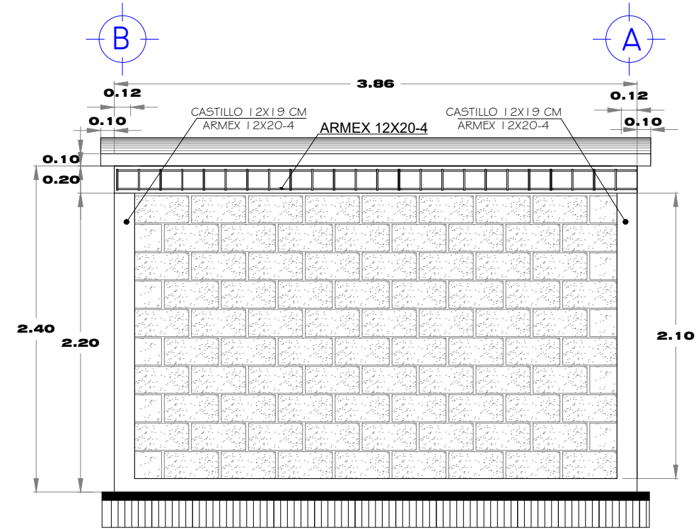
ALZADO POSTERIOR
