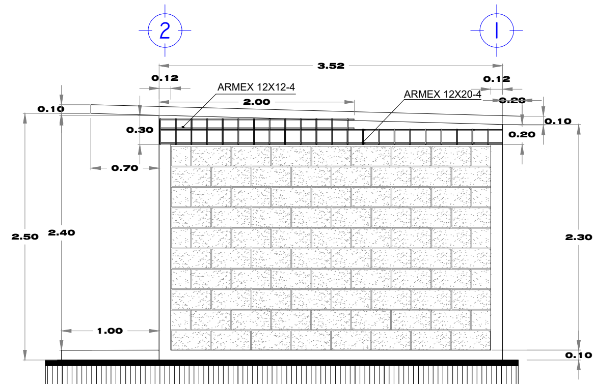
ALZADO LATERAL
