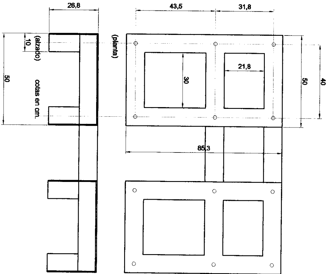
(BASE PARA COLOCACION DE MOTORES DE PROCESO)
