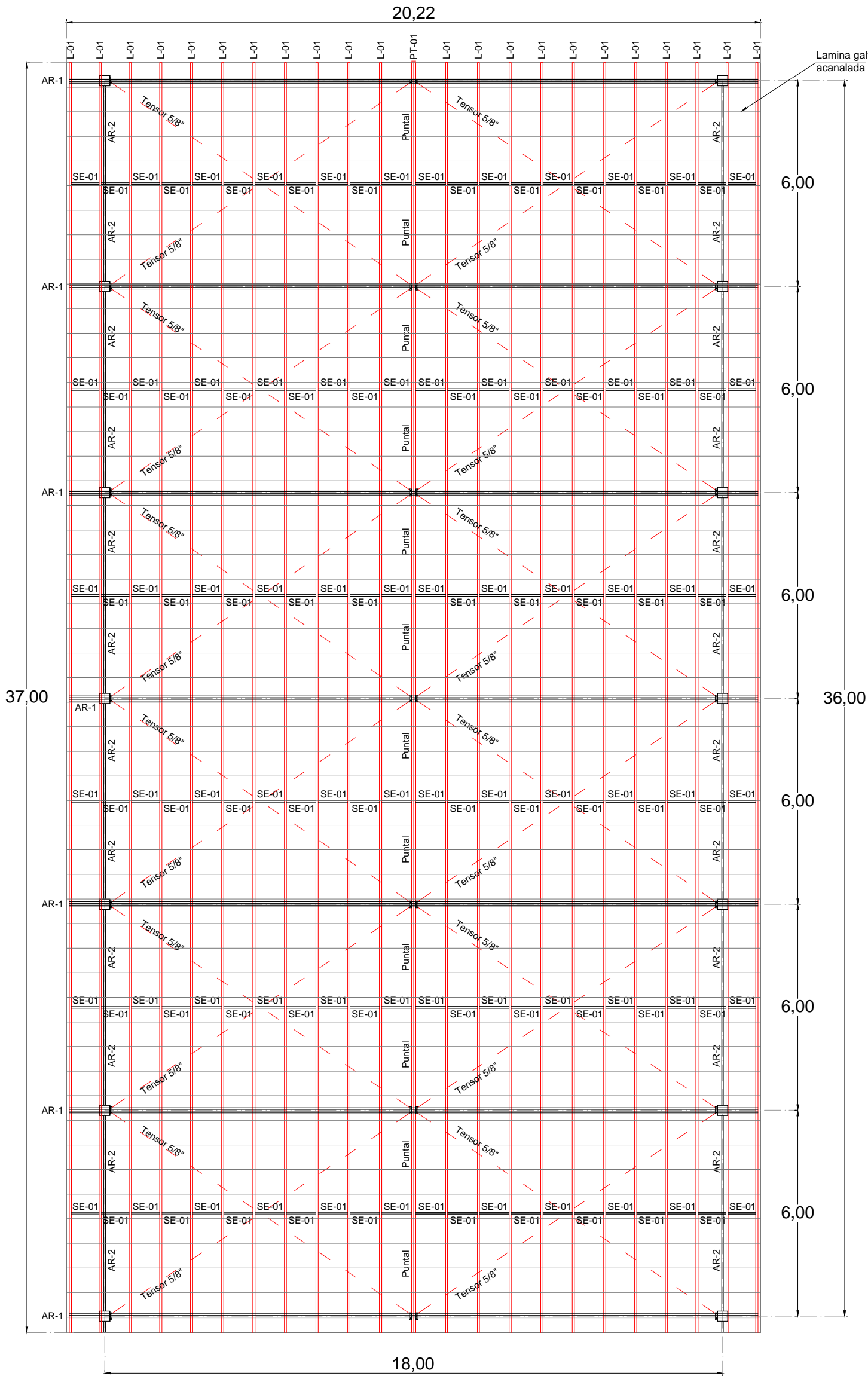
PLANTA ESTRUCTURAL DE CUBIERTA
