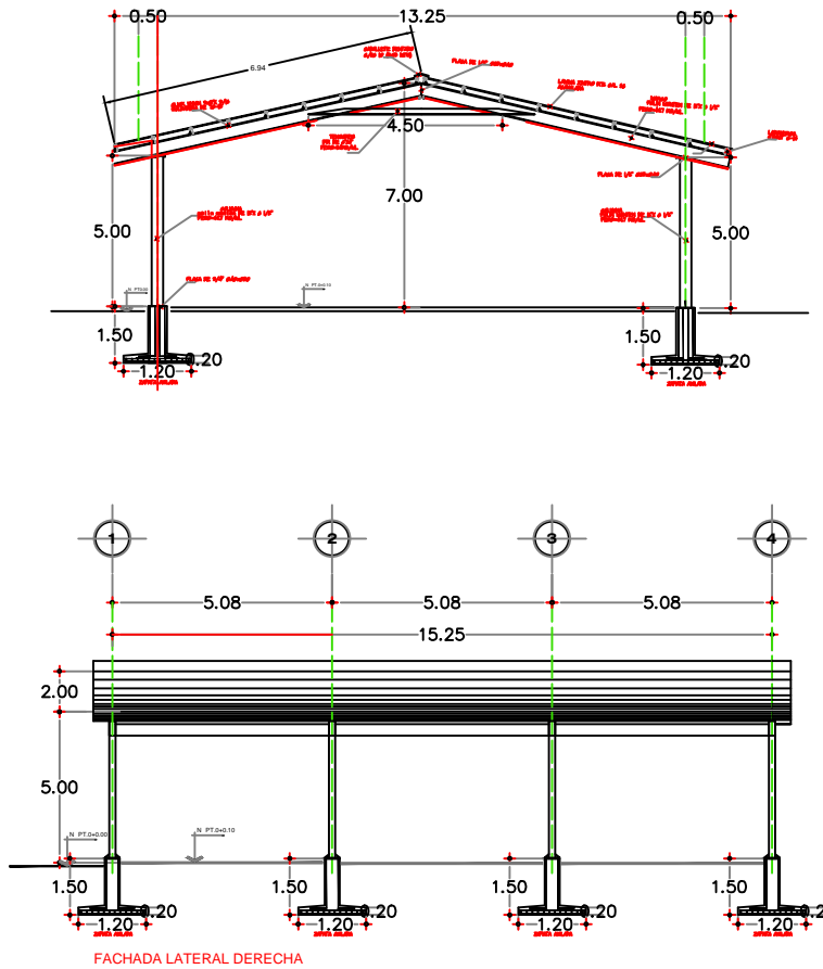
FACHADA LATERAL DERECHA
