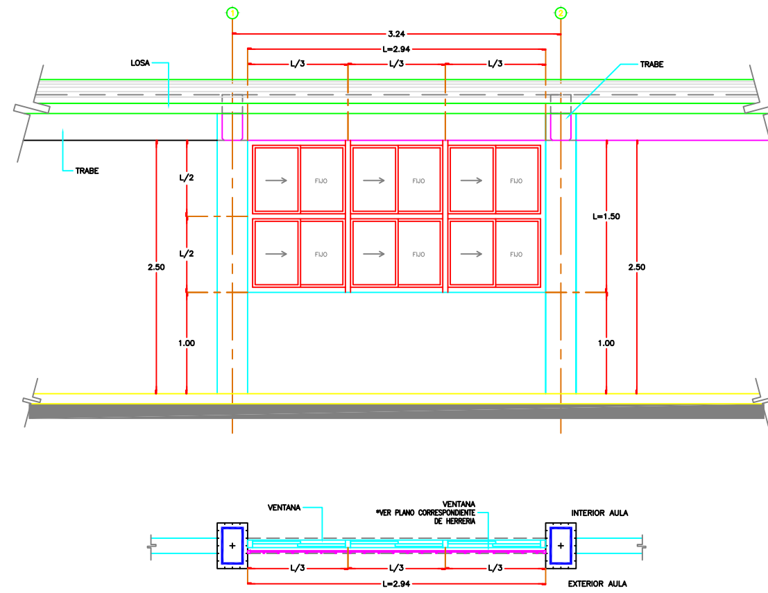
2 CANCELERIA EN FACHADA POSTERIOR – MUROS BAJOS
