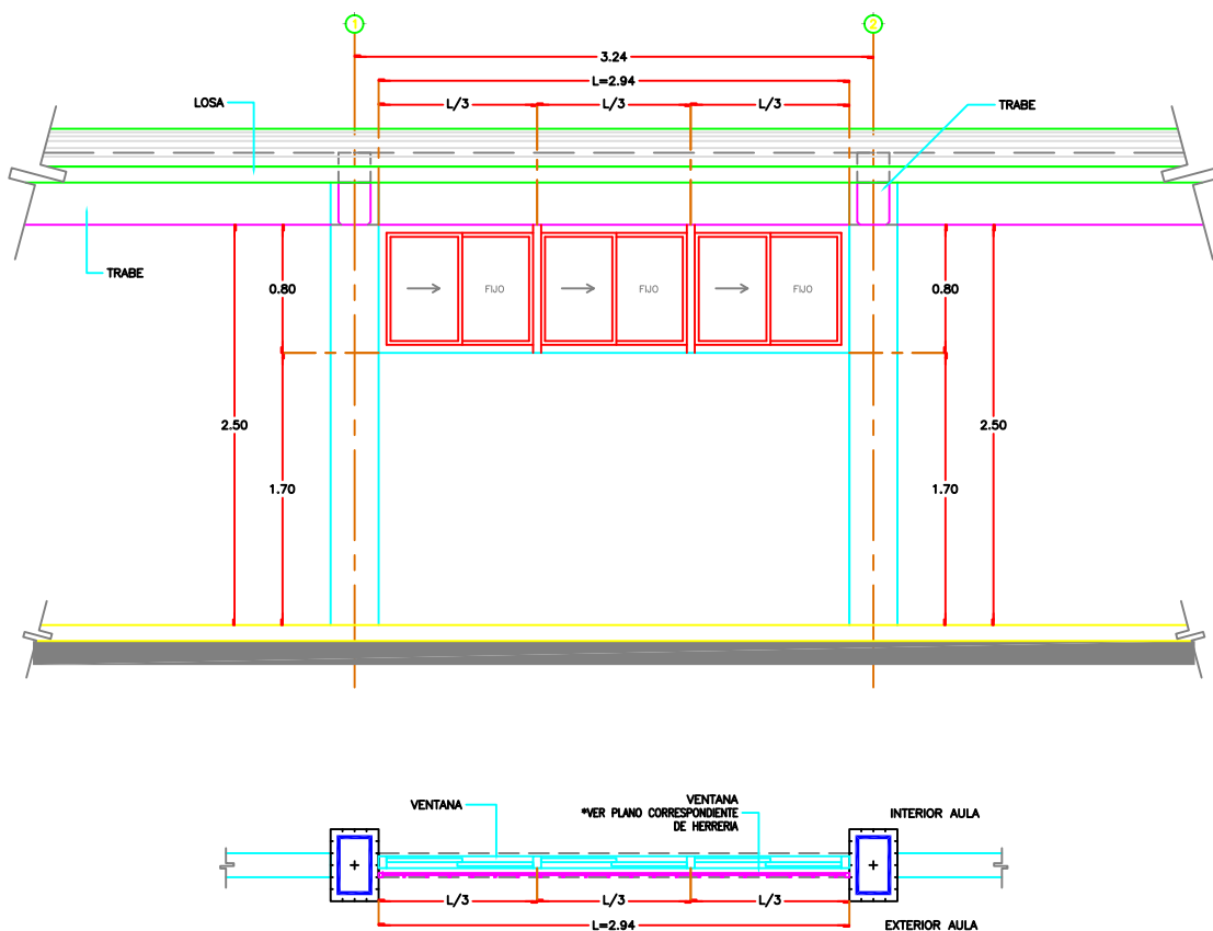
4 CANCELERIA EN FACHADA POSTERIOR – MUROS ALTOS
