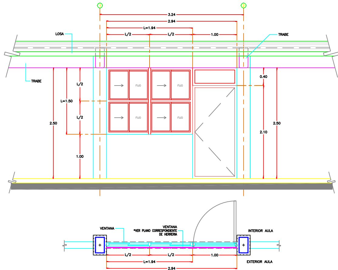
1 CANCELERIA EN FACHADA PRINCIPAL – MUROS BAJOS
