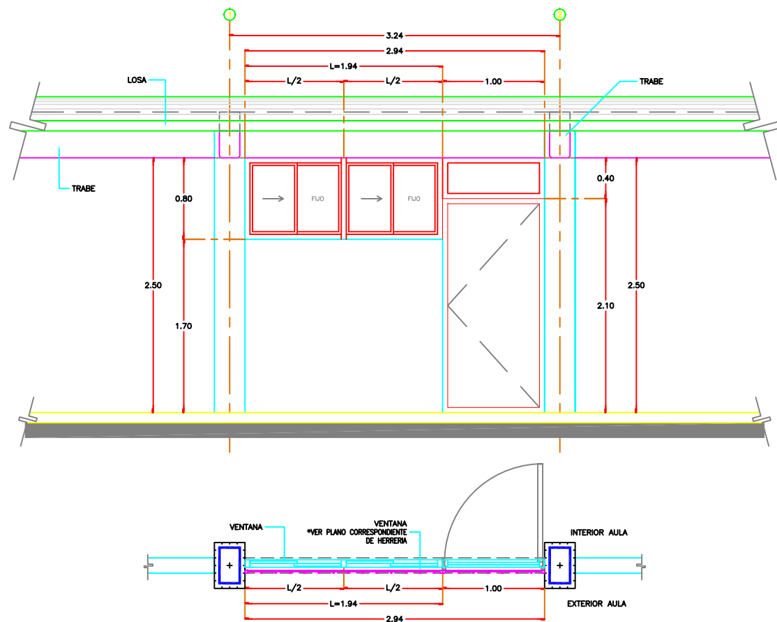
3 CANCELERIA EN FACHADA PRINCIPAL – MUROS ALTOS
