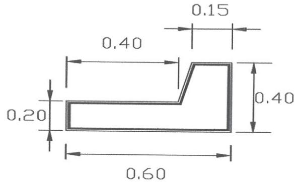
DETALLE DE GUARNICION TIPO "L"
