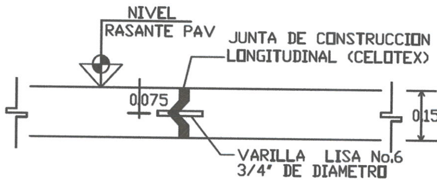
DETALLE DE JUNTA CONSTRUCTIVA (VISTA PARALELA AL EJE DE CALLE)
