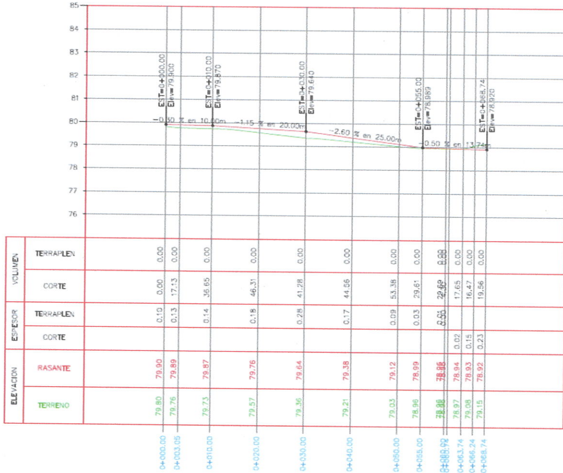
PLANTA DE PERFIL
