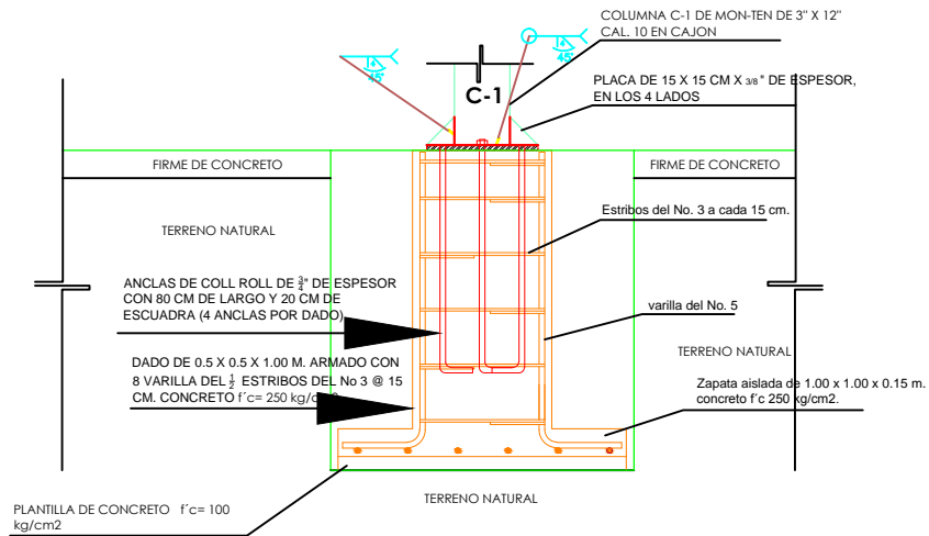
Detalle Z-1
