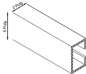
LARGUERO TIPO MON-TEN 5" x 2" CAL 12 SOLDADO A TRABE
