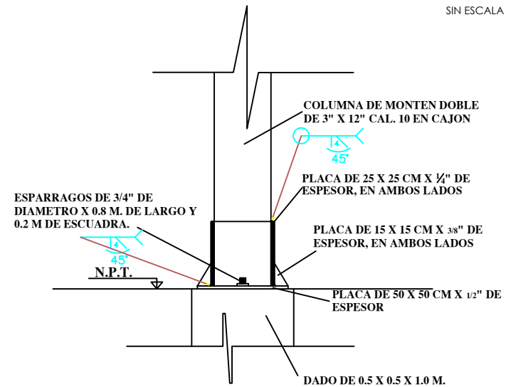
Detalle CONEXIÓN DADO Y MONTEN
