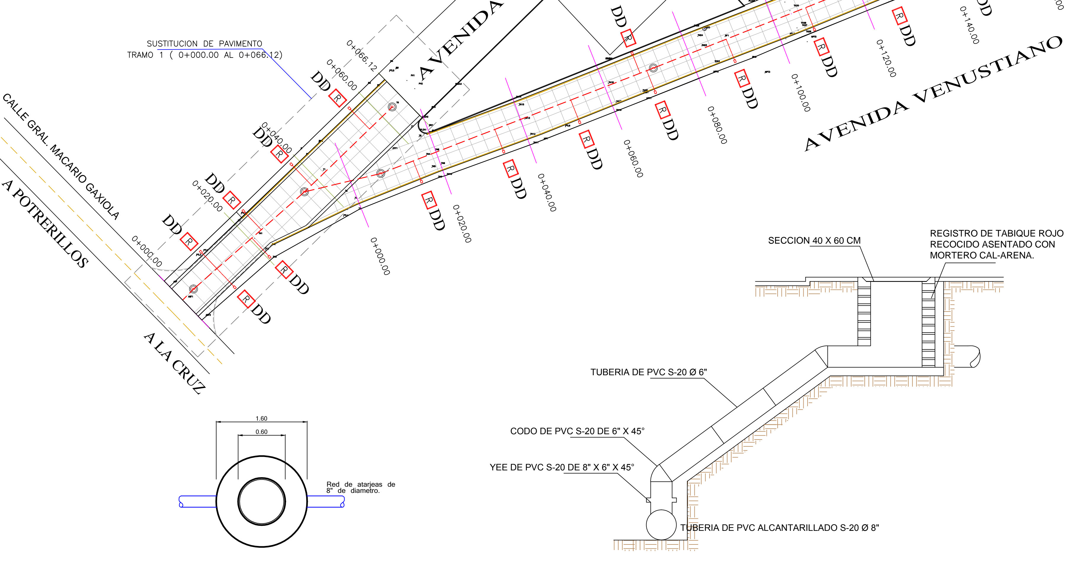
Planta de Pozos de visita.- Sin escala.-
