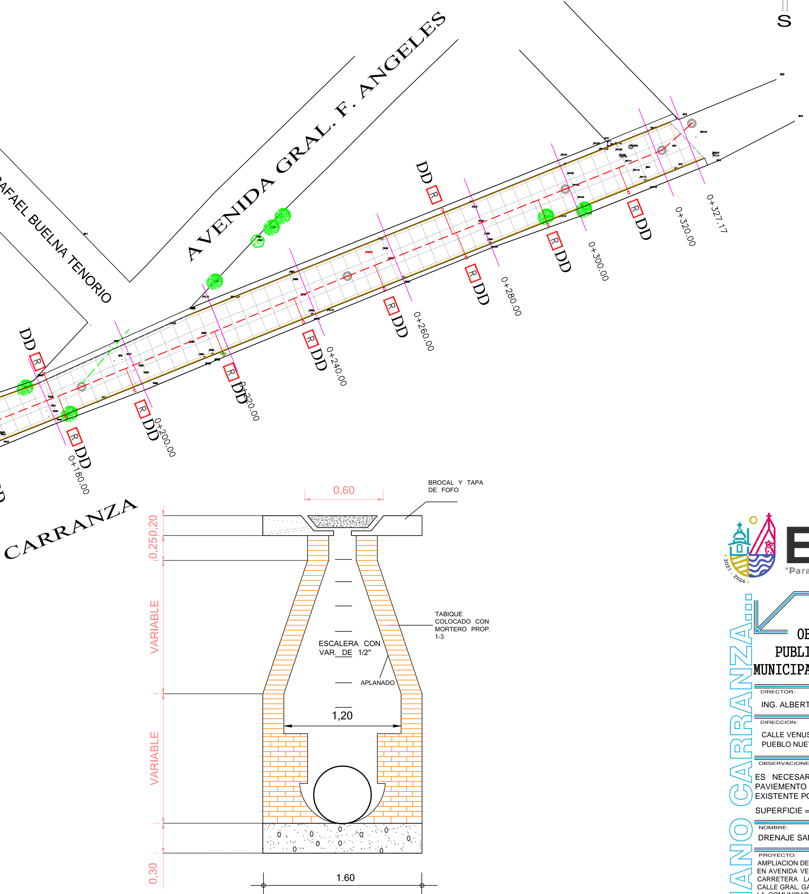
Detalle de Pozos de visita.- Sin escala.-
