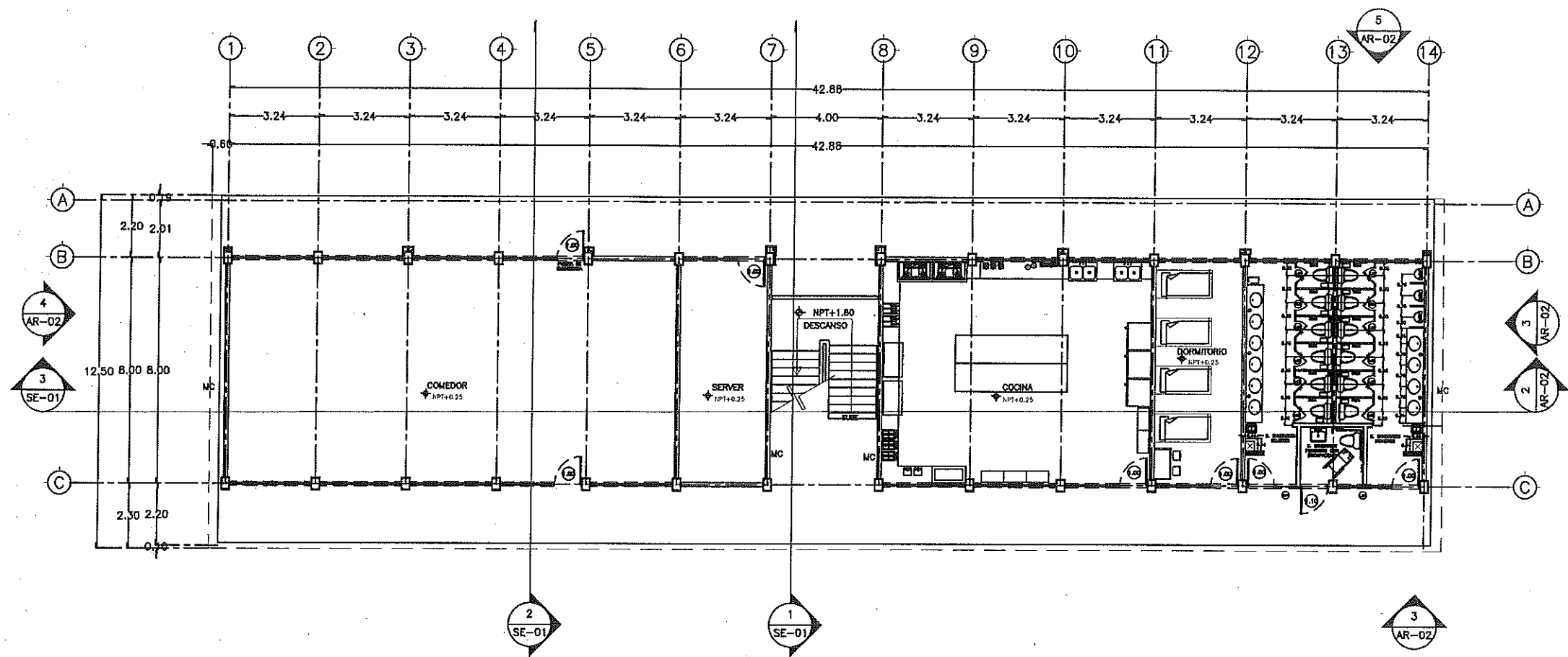
PLANTA ARQUITECTONICA BAJA
