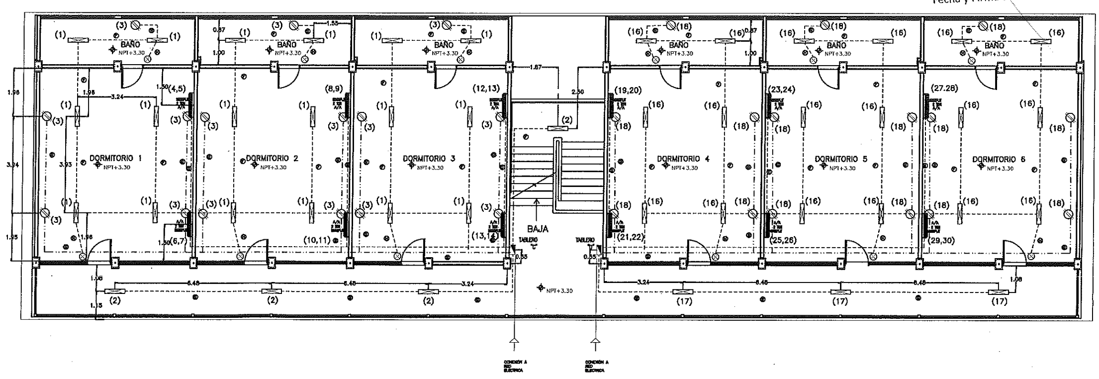
2 INSTALACION ELECTRICA PLANTA ALTA
