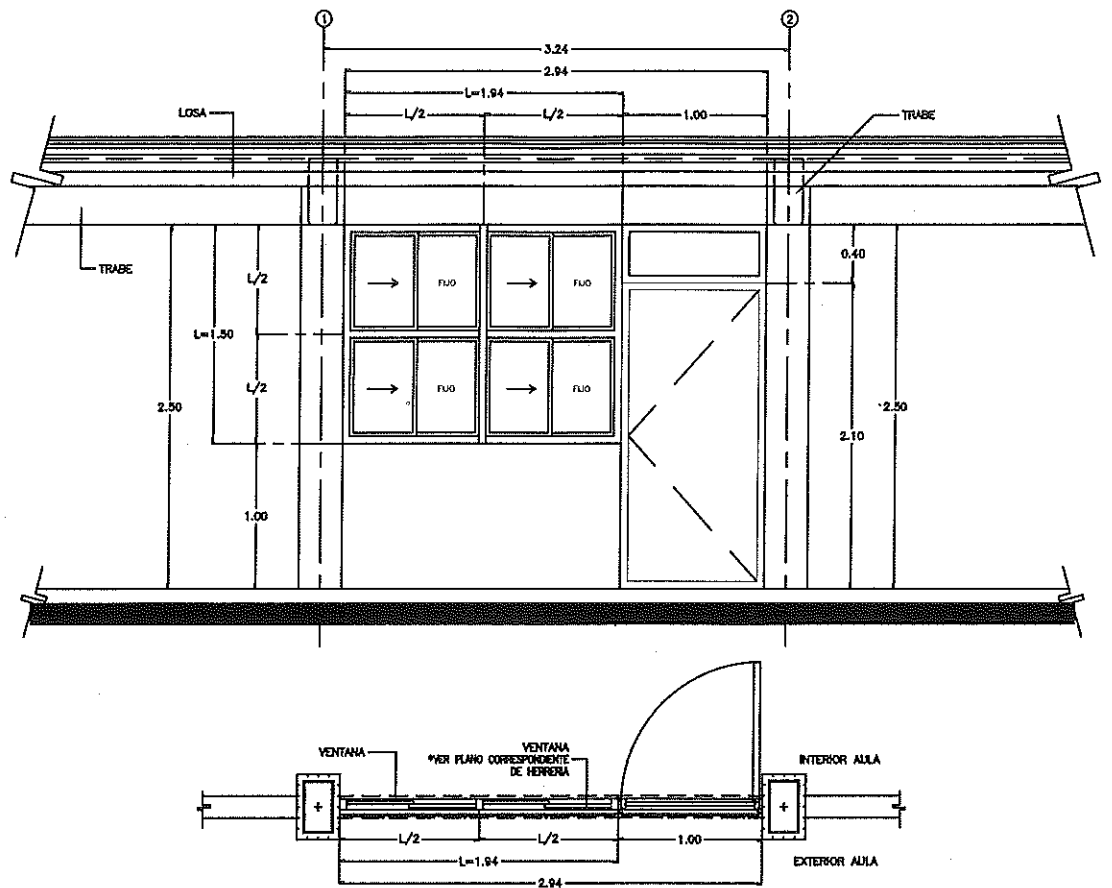
1 CANCELERIA EN FACHADA PRINCIPAL - MUROS BAJOS ESC.1:50
