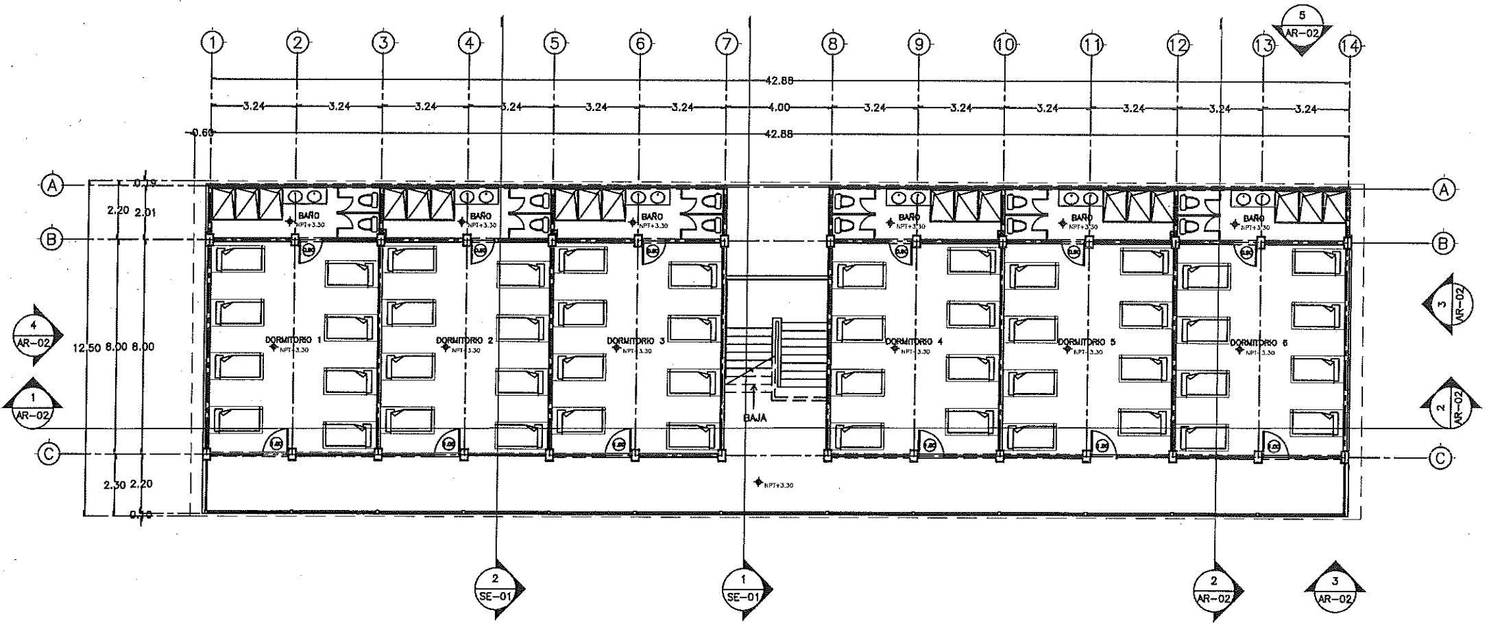
PLANTA ARQUITECTONICA ALTA
