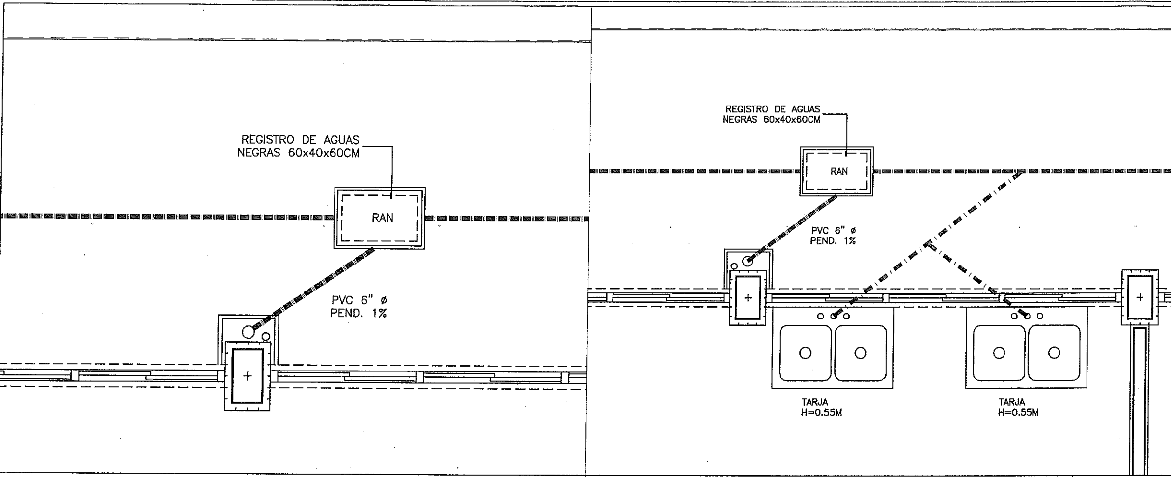
DETALLE - CONEXIÓN A R.A.N.
