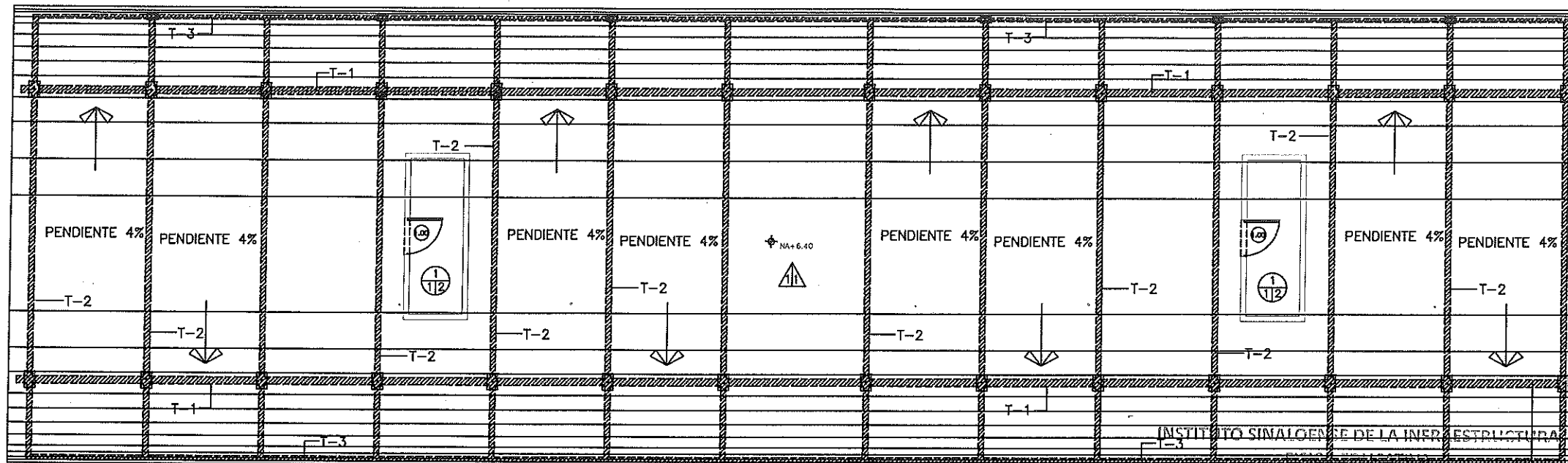
1 PLANTA DE AZOTA Proyecto Autorizado de la Obra No. 230001 ESC. 1:75 PGO. No. 23101 por el Departamento de Proyectos y Certificación.
