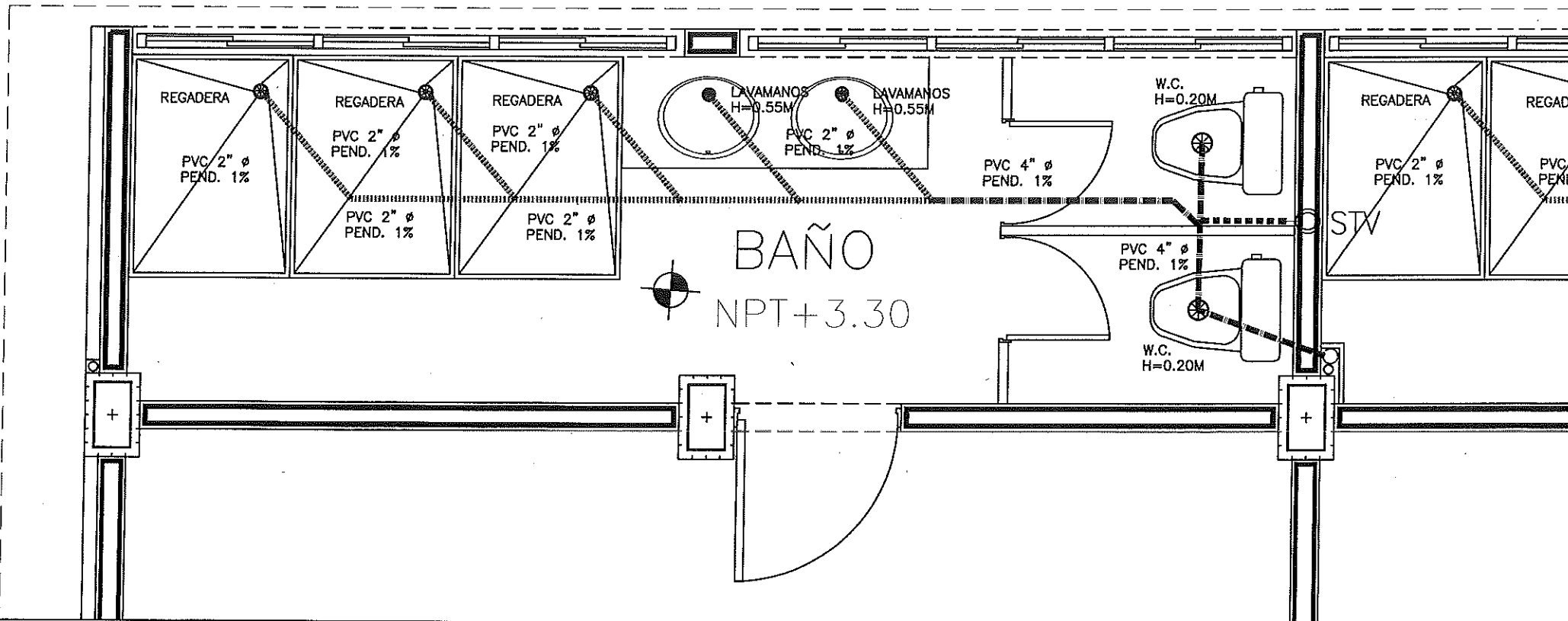
DETALLE - BAÑO DE DORMITORIOS
