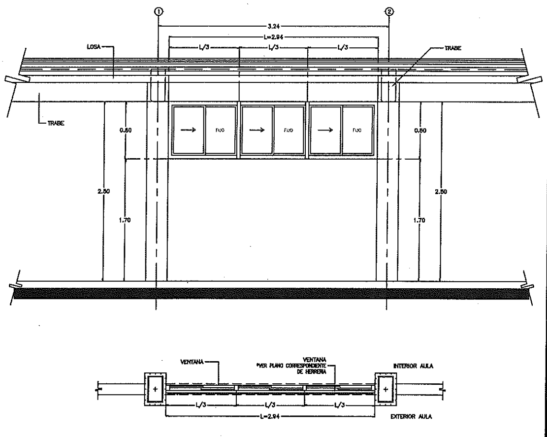
4 CANCELERIA EN FACHADA POSTERIOR - MUROS ALTOS ESC.1:50
