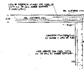
DETALLE DE ARMADO DE LOSA Y MURO SIN ESCALA
