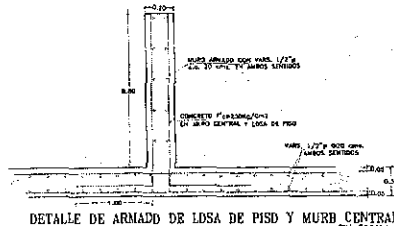
DETALLE DE ARMADO DE LOSA DE PISO Y MURO CENTRAL SIN ESCALA
