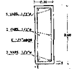
DETALLE DE TRABE T-2 SIN ESCALA
