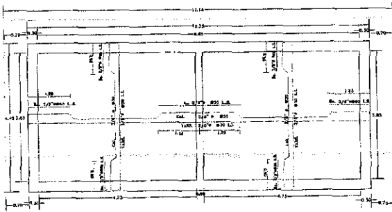
DETALLE DE ARMADO DE LOSA SUPERIOR SIN ESCALA
