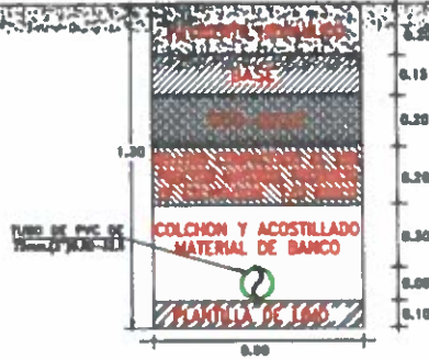
SECCIÓN DE ZANJA PARA TUBERÍA DE 3 º . EN PAVIMENTO
