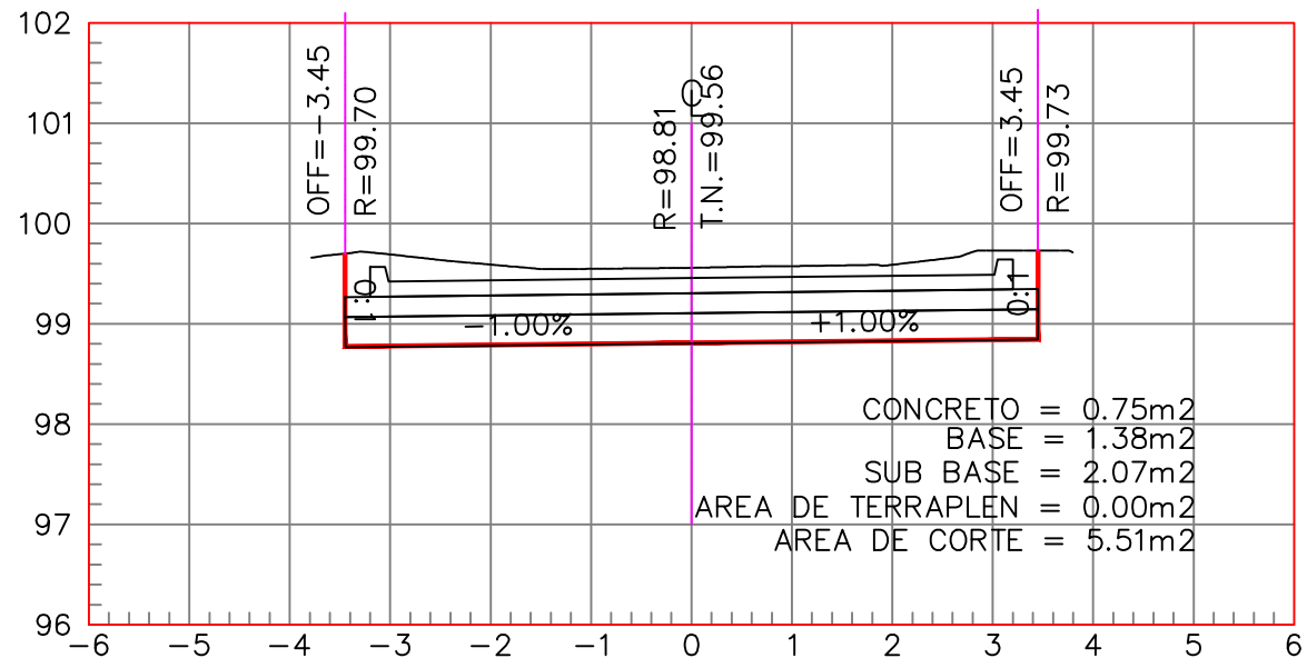
ESTACION 0+080.00 ESCALA HORIZONTAL 1 : 100 ESCALA VERTICAL 1 : 100
