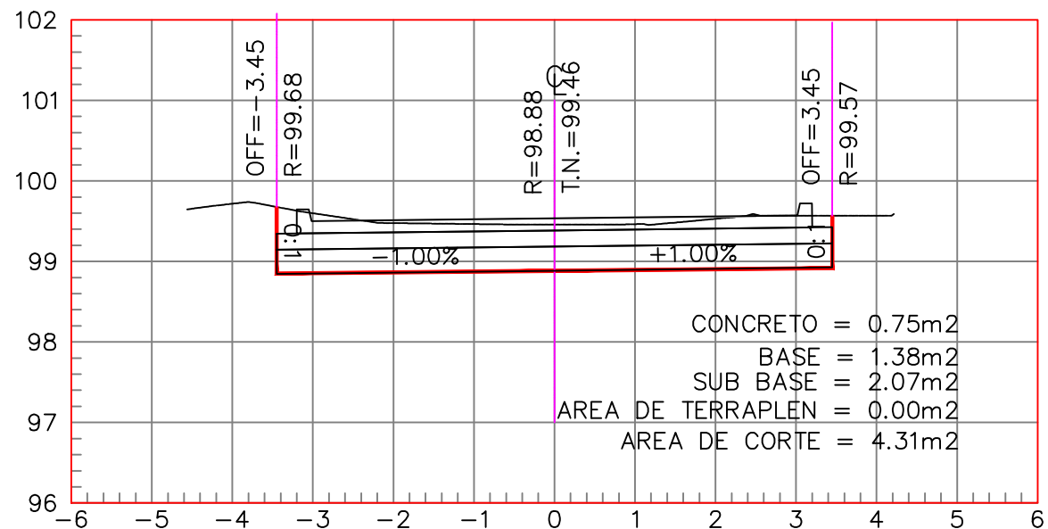
ESTACION 0+100.00 ESCALA HORIZONTAL 1 : 100 ESCALA VERTICAL 1 : 100
