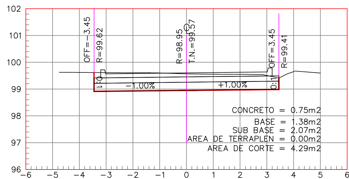
ESTACION 0+117.64 ESCALA HORIZONTAL 1 : 100 ESCALA VERTICAL 1 : 100
