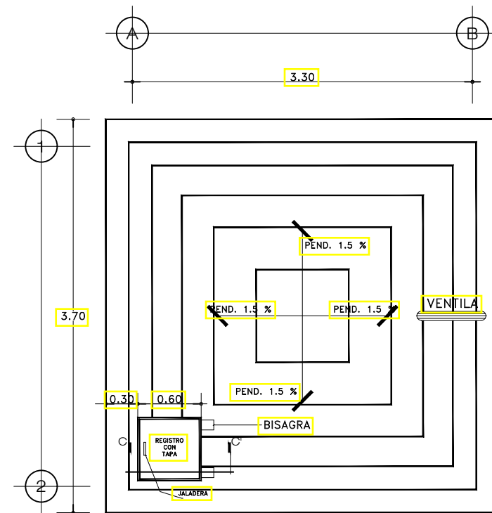
PLANTA DE AZOTEA ESC. 1:50
