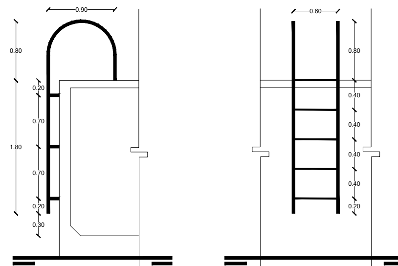
DETALLE ESCALERA ESC. 1:50
