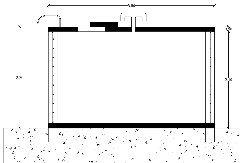
CORTE (A) ESC. 1:50
