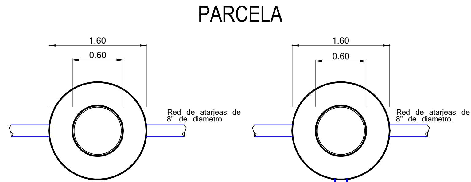
Planta de Pozos de visita.- Sin escala.-
