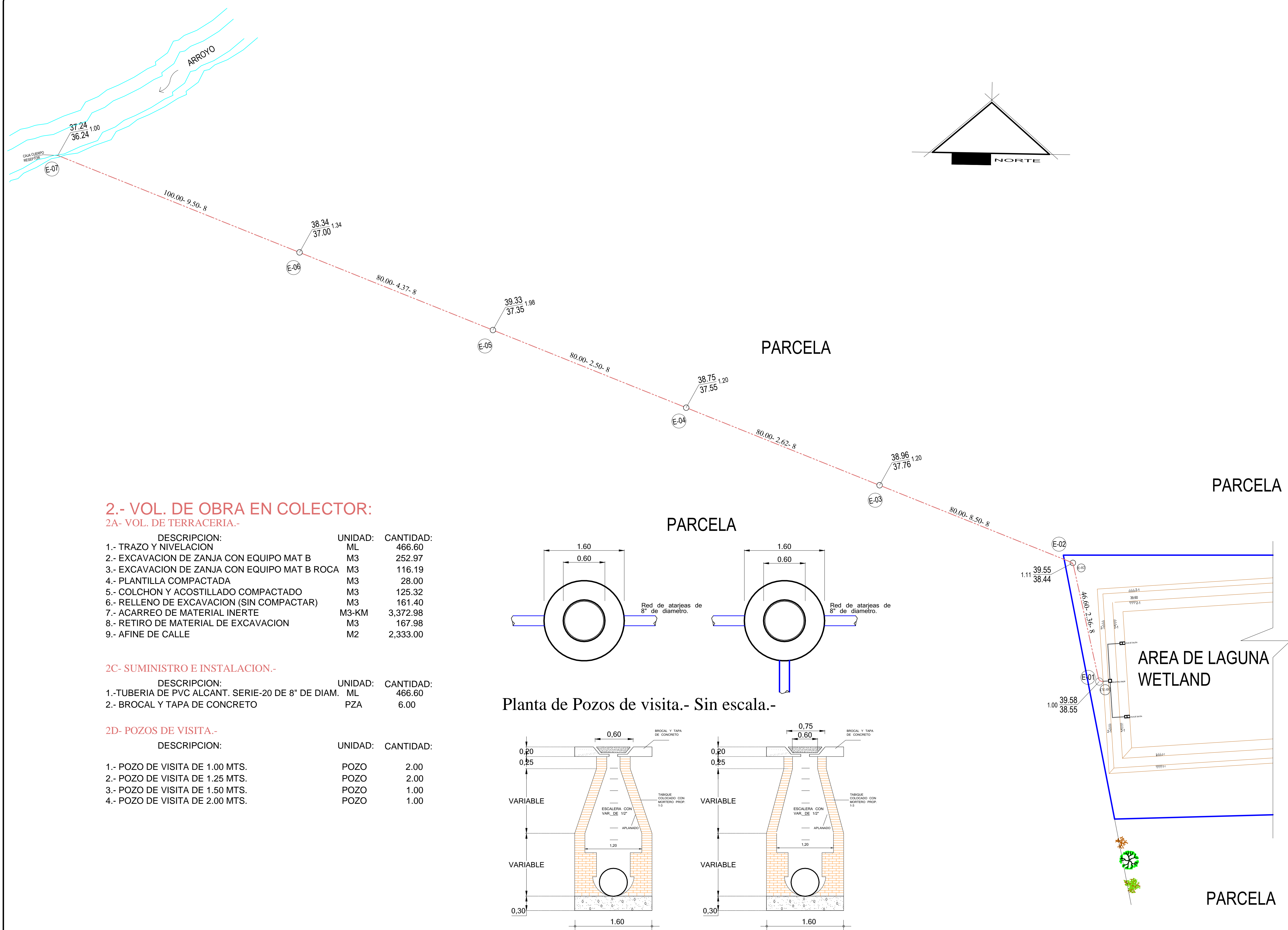
DETALLE DE POZO DE VISTA.- Sin escala.-
