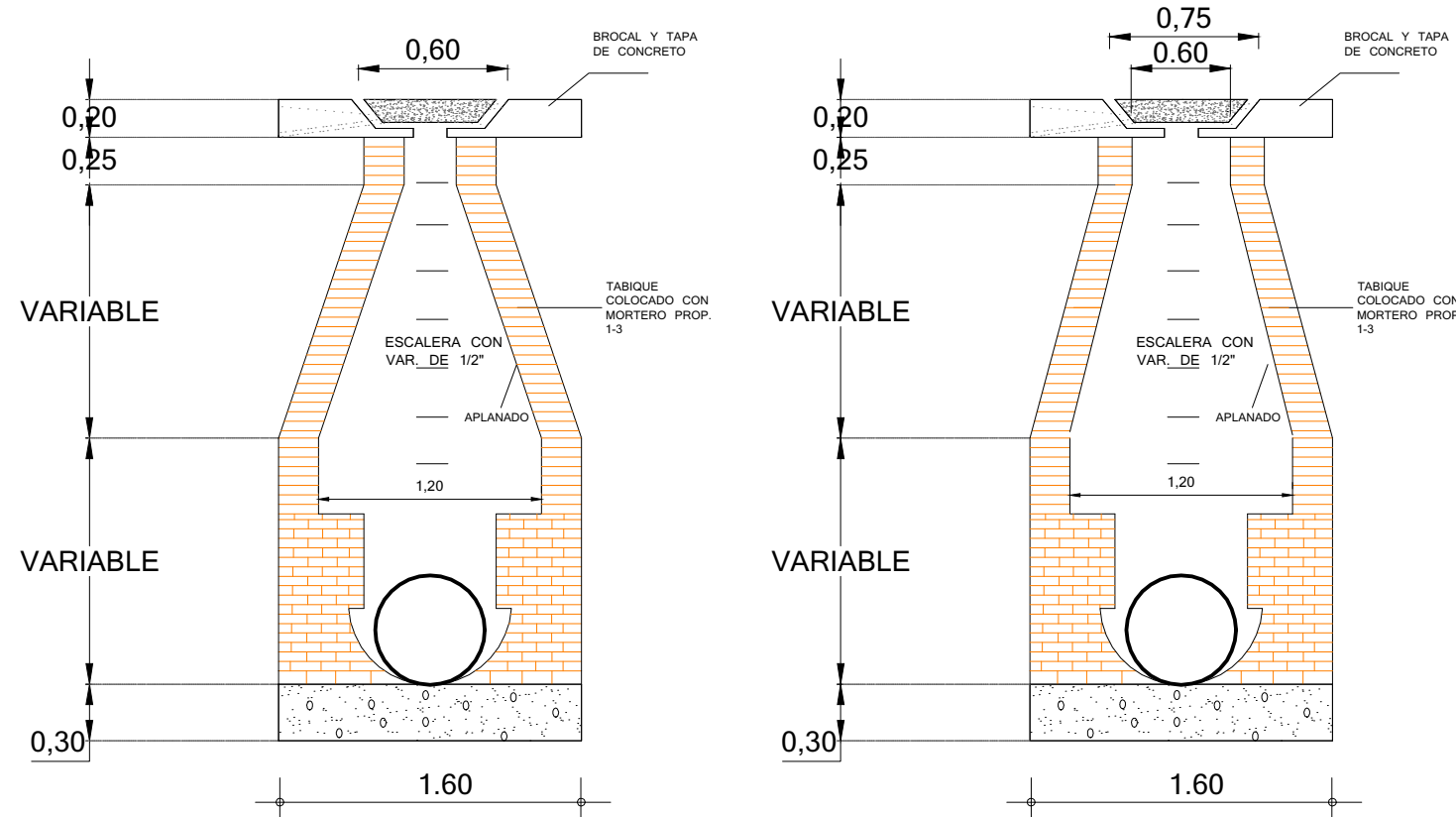
DETALLE DE POZO DE VISTA.- Sin escala.-
