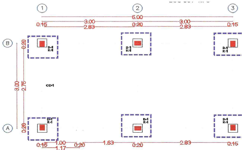
PLANTA DE DADOS DE CIMENTACION
