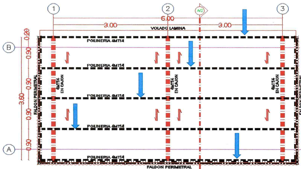
PLANTA DE TECHUMBRE
