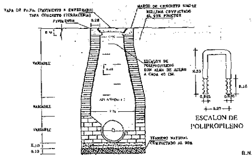
CORTE A-A POZO DE VISITA COMUN
