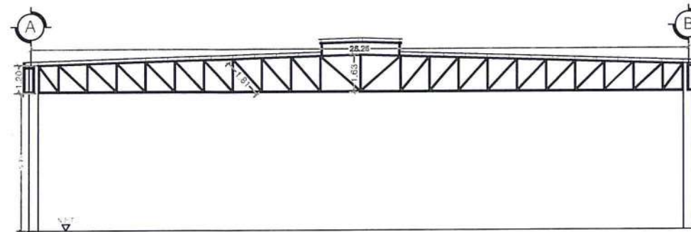
2 ALZADO ESTRUCTURAL SIN ESCALA
