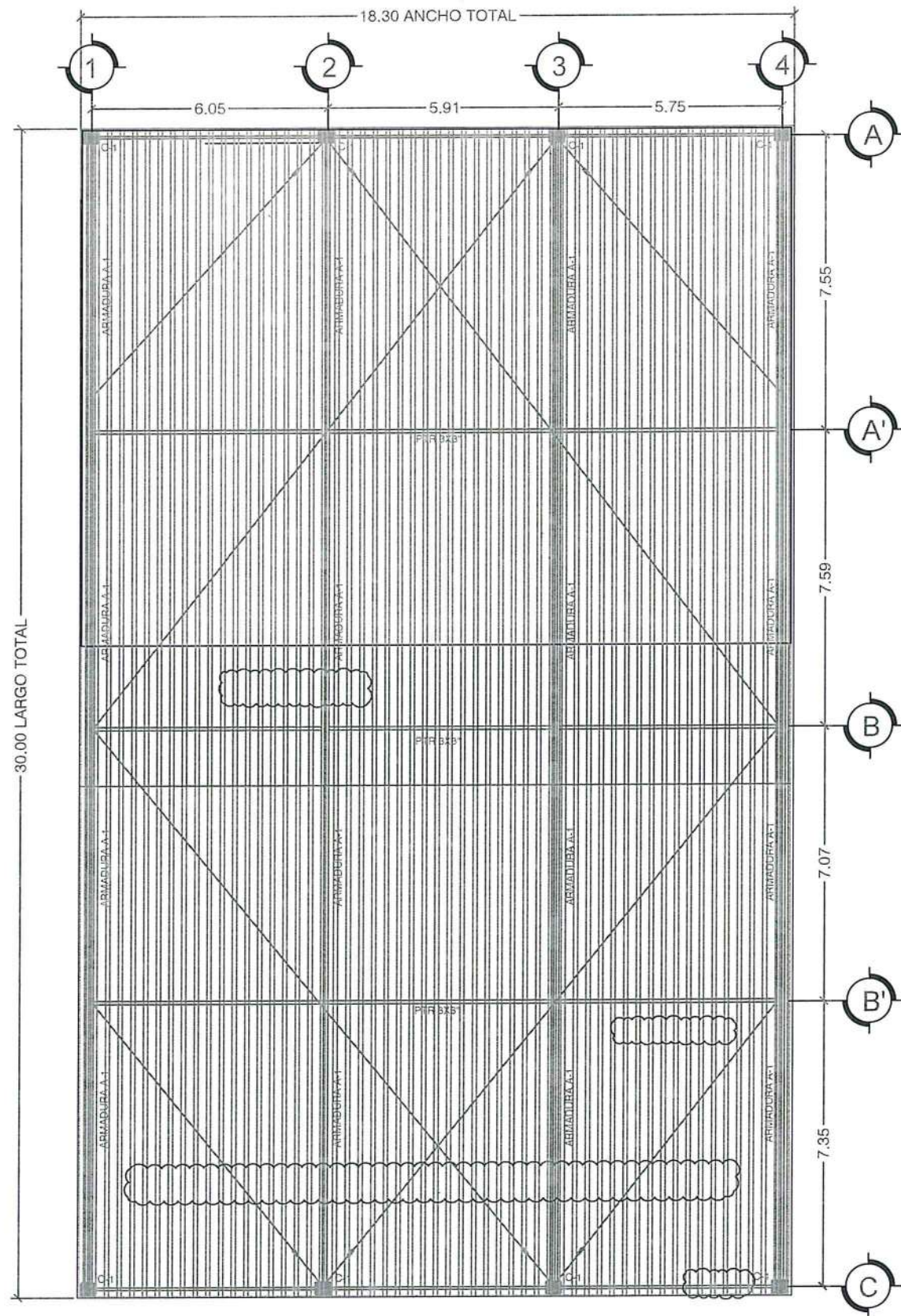
1 PLANTA DE ESTRUCTURA SIN ESCALA
