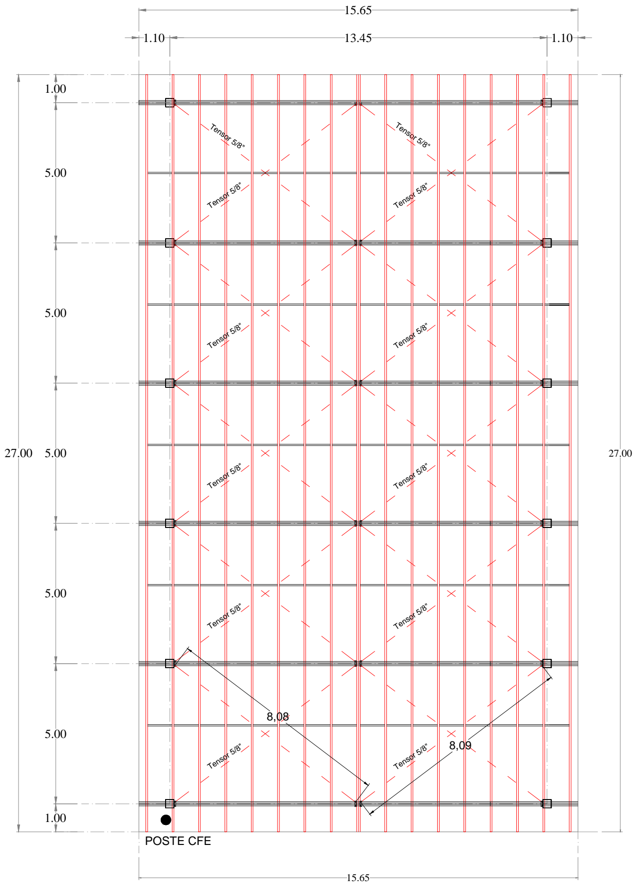
PLANTA ESTRUCTURAL
