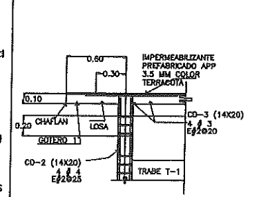
CORTE F-F
