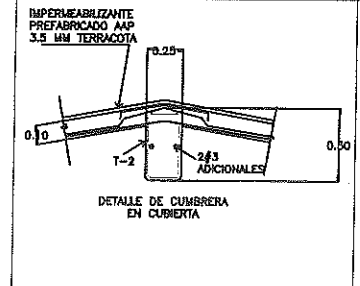
CORTE X-X
