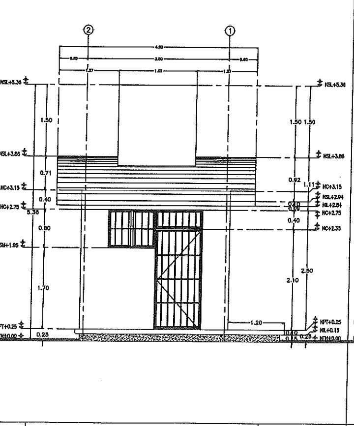
3 ALZADO PRINCIPAL ESC, 1:75
