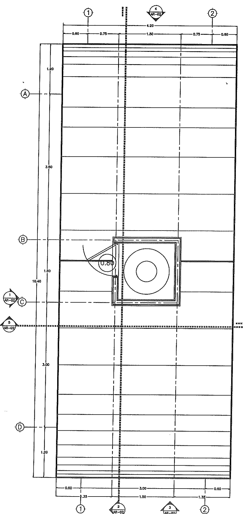
2 PLANTA DE AZOTEA ESC, 1:50
