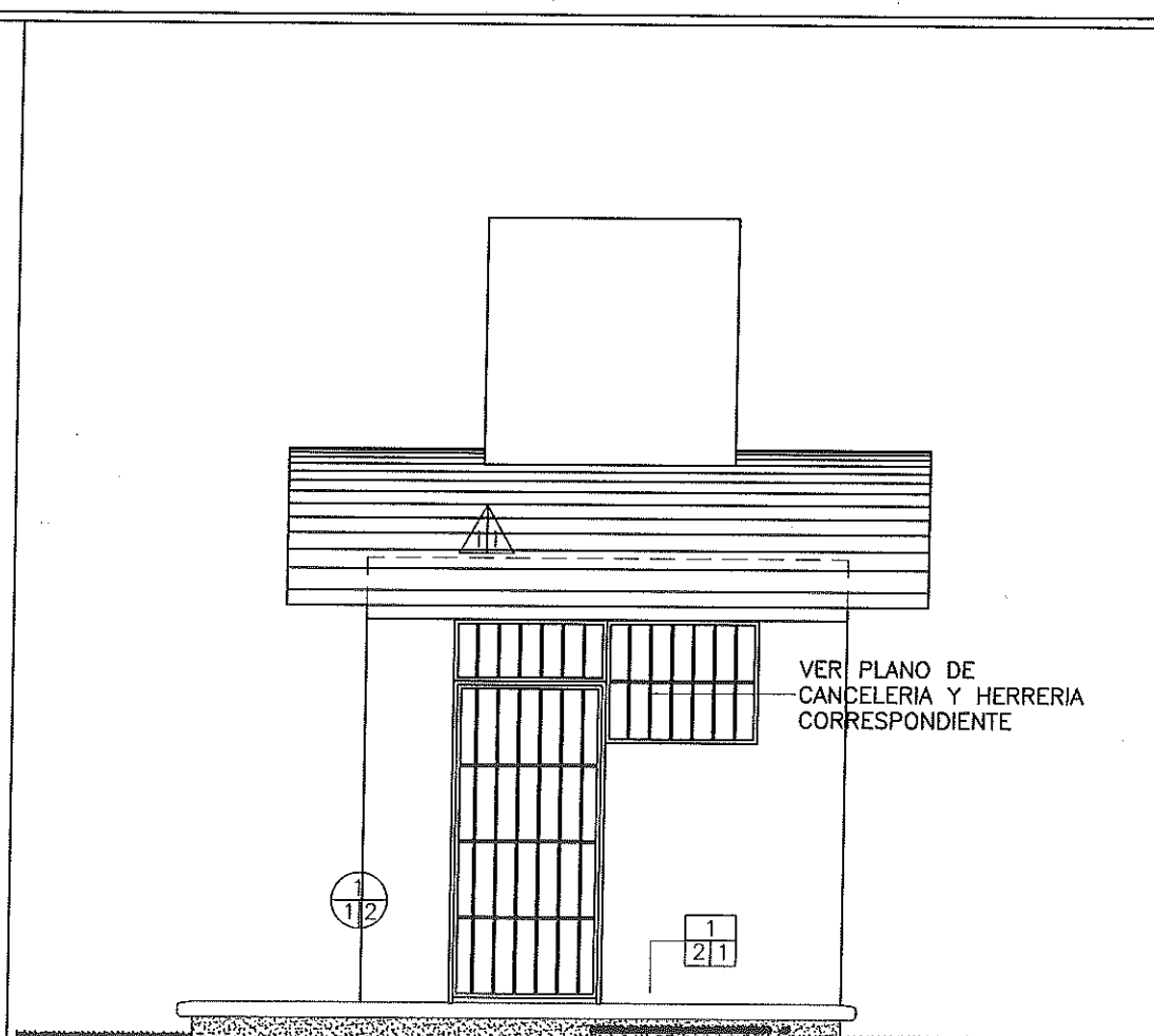
2 ALZADO POSTERIOR ESC, 1:100
