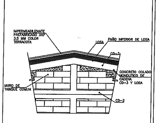
DETALLE DE MURO CABECERO
