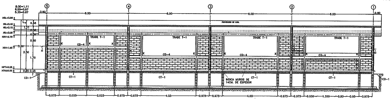
FACHADA ESTRUCTURAL POSTERIOR
