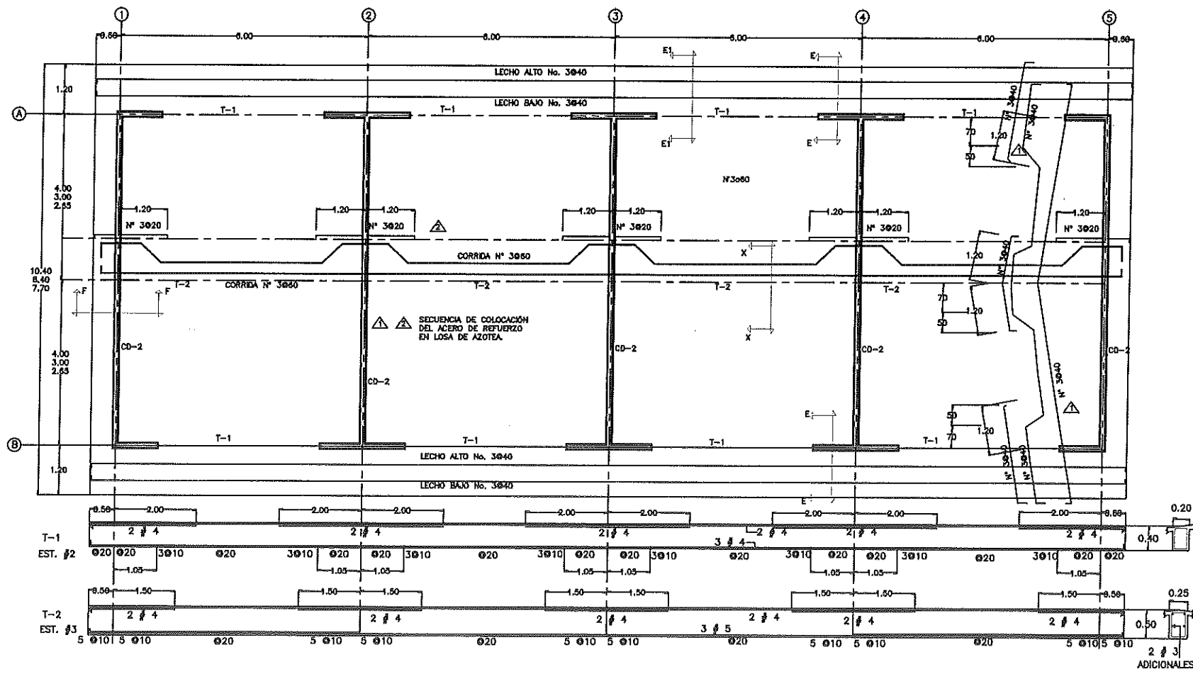
PLANTA DE ARMADO DE LOSA (AGRUPAMIENTO MAXIMO 4 AULAS)
