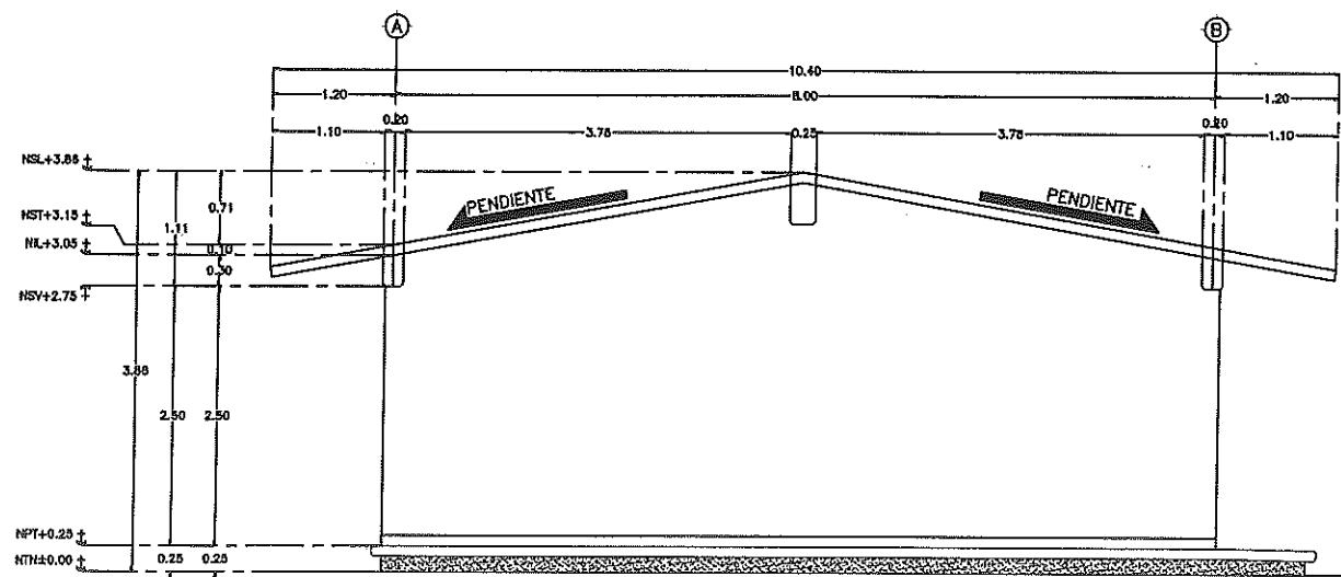
FACHADA LATERAL
