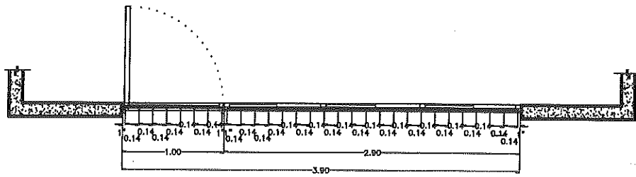
1 HERRERIA EN FACHADA PRINCIPAL – TALLERES Y LABORATORIOS ESC. 1:50
