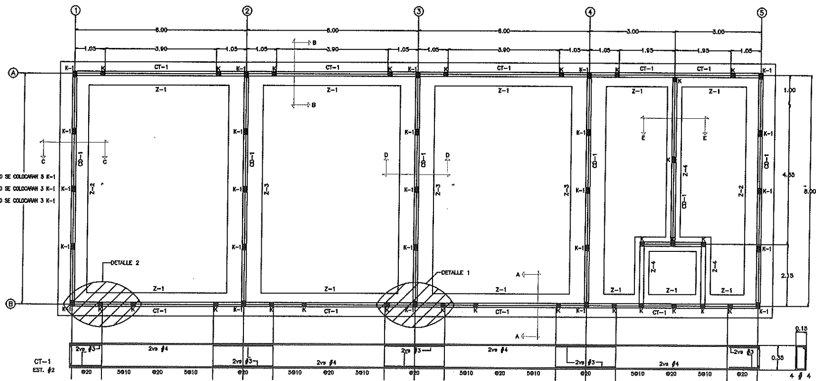
PLANTA DE CIMENTACIÓN (AGRUPAMIENTO MAXIMO 4 AULAS) ESC. 1:25
