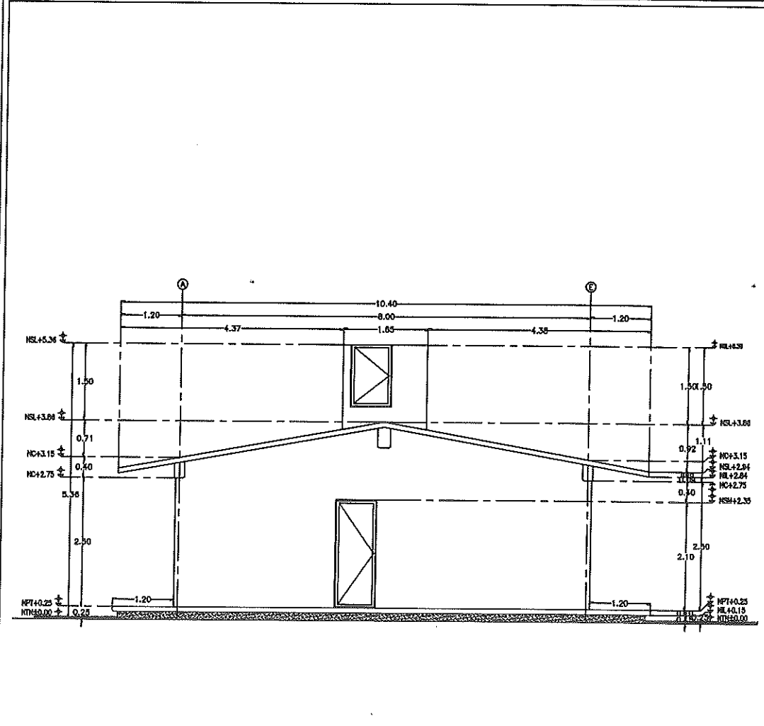
1 ALZADO LATERAL ESC, 1:100
