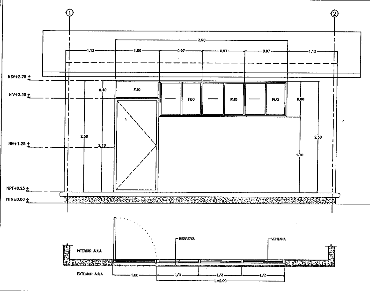
1 C. EN FACHADA PRINCIPAL-TALLERES Y LABORATORIOS ESC. 1:50
