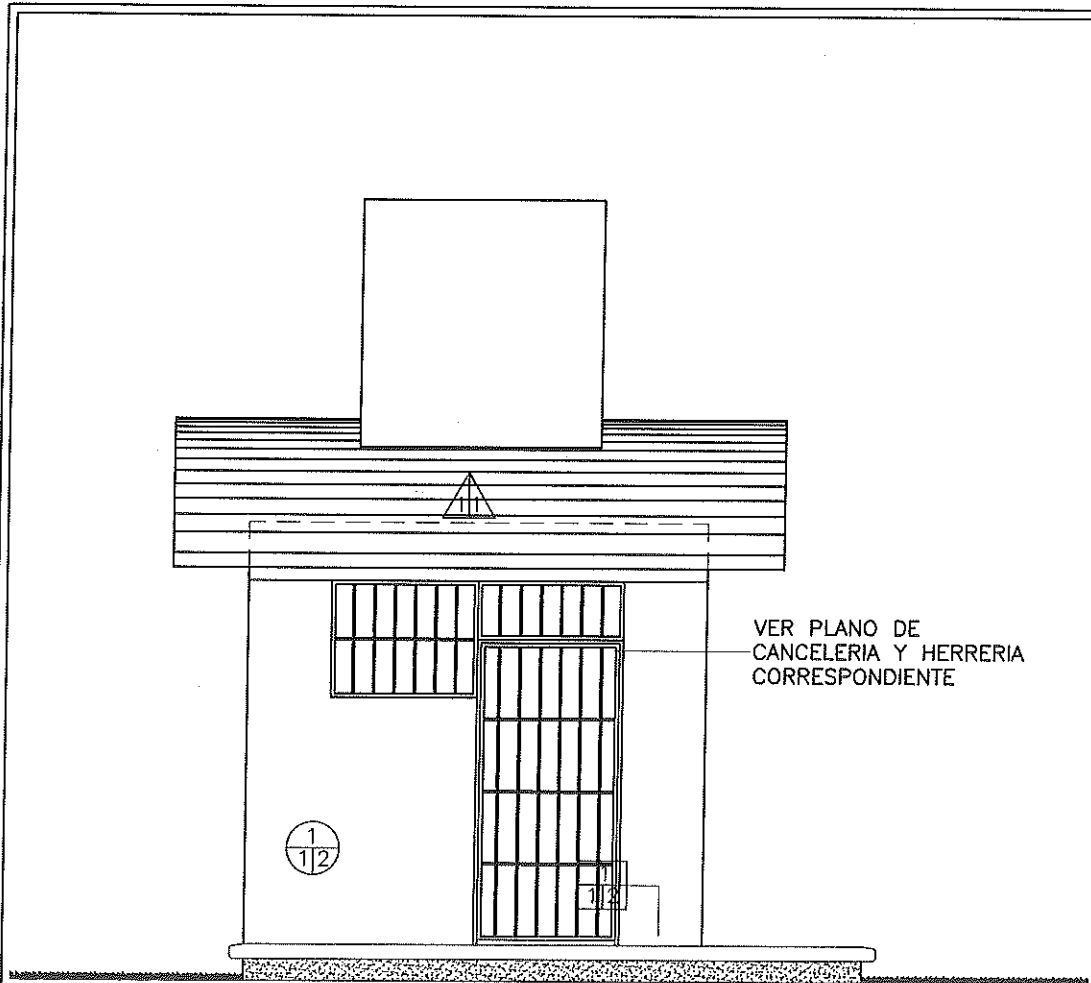
1 ALZADO PRINCIPAL ESC, 1:100
