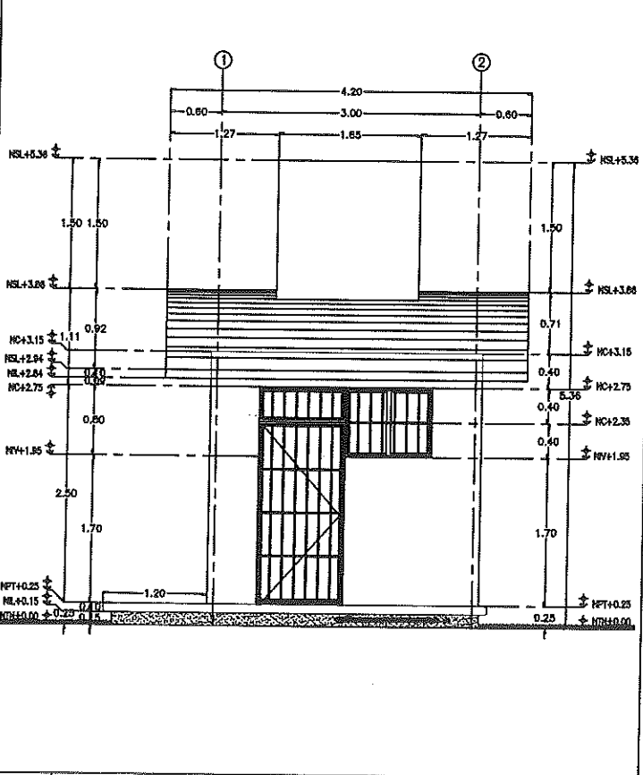
4 ALZADO POSTERIOR ESC, 1:75
