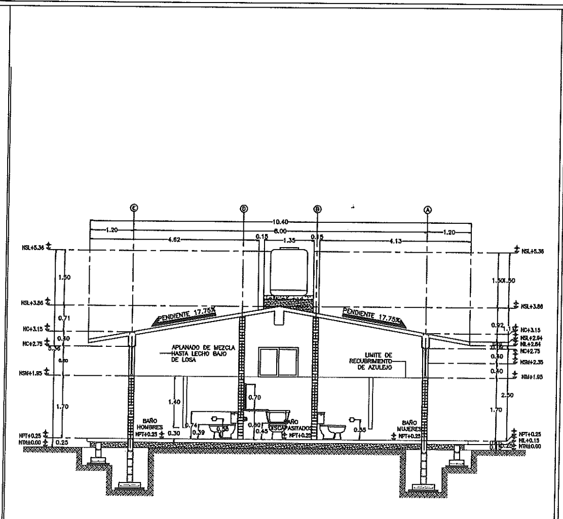
2 SECCIÓN LONGITUDINAL ESC, 1:100
