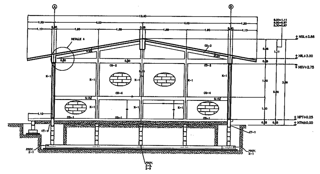
CORTE ESTRUCTURAL TRANSVERSAL
