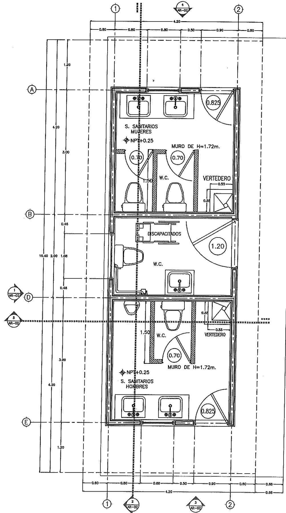
1 PLANTA ARQUITECTONICA ESC, 1:50
