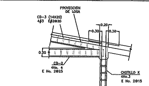
DETALLE 4
