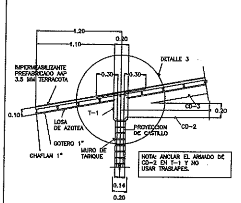
CORTE E-E
