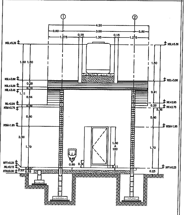
5 SECCIÓN TRANSVERSAL ESC, 1:75
