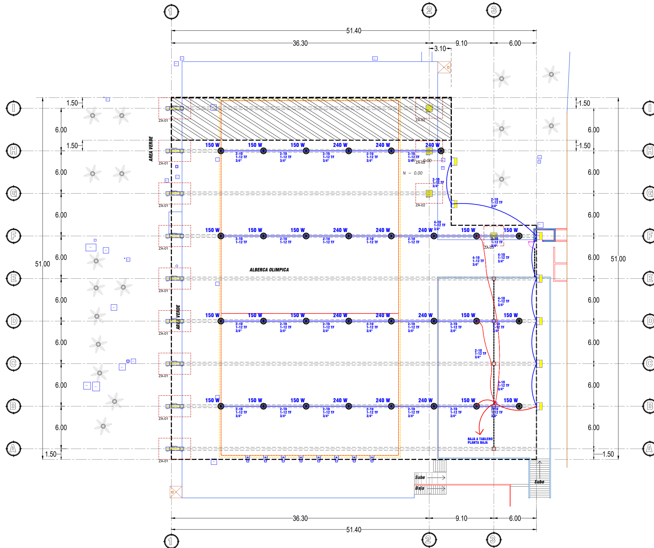
PLANTA ARQUITECTÓNICA
